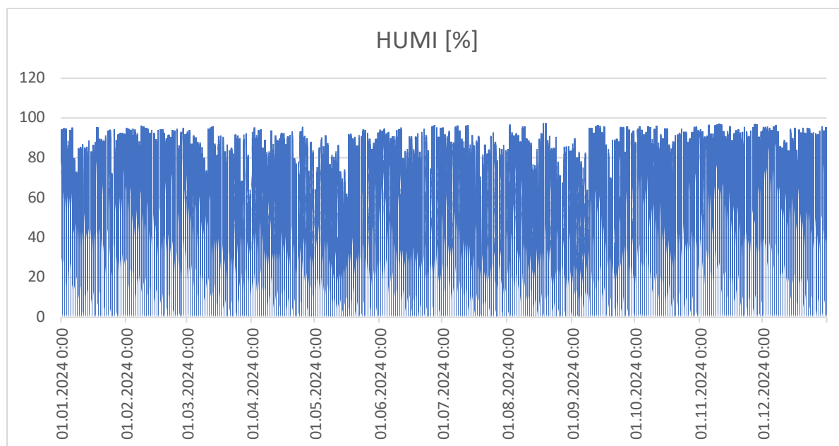
Obr. 16: Vývoj relativní vlhkosti na stanici 2524, včetně trendu.
