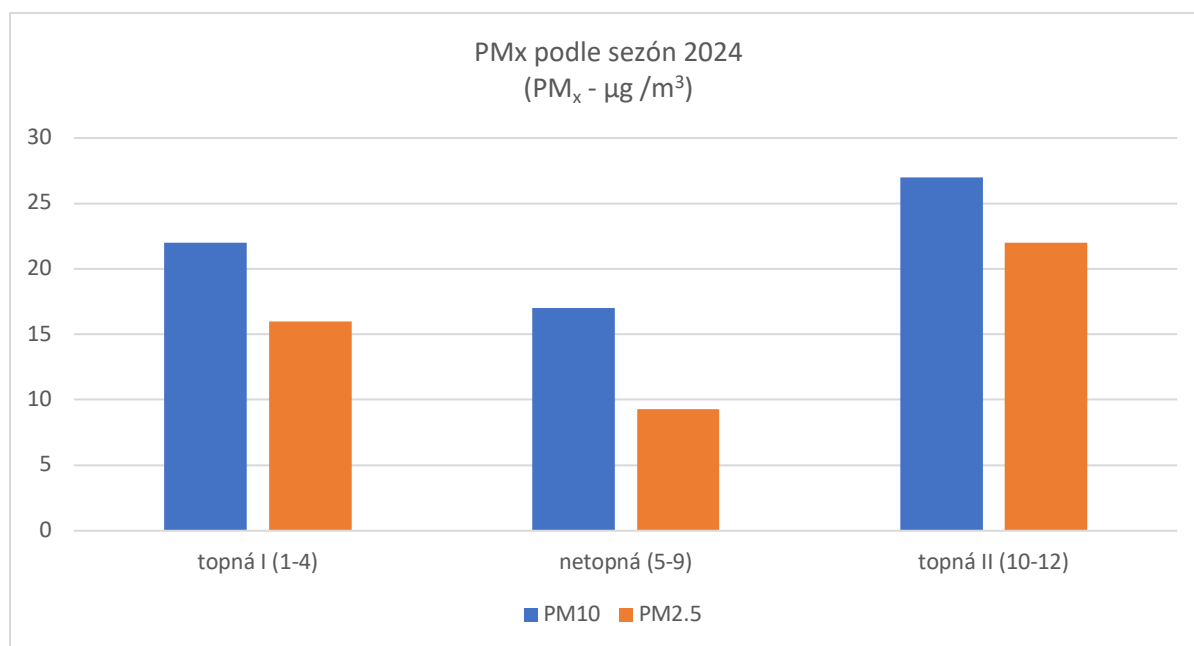
Obr. 3: Porovnání průměrných hodnot PM_x podle sezón na stanici 2524 v roce 2024
