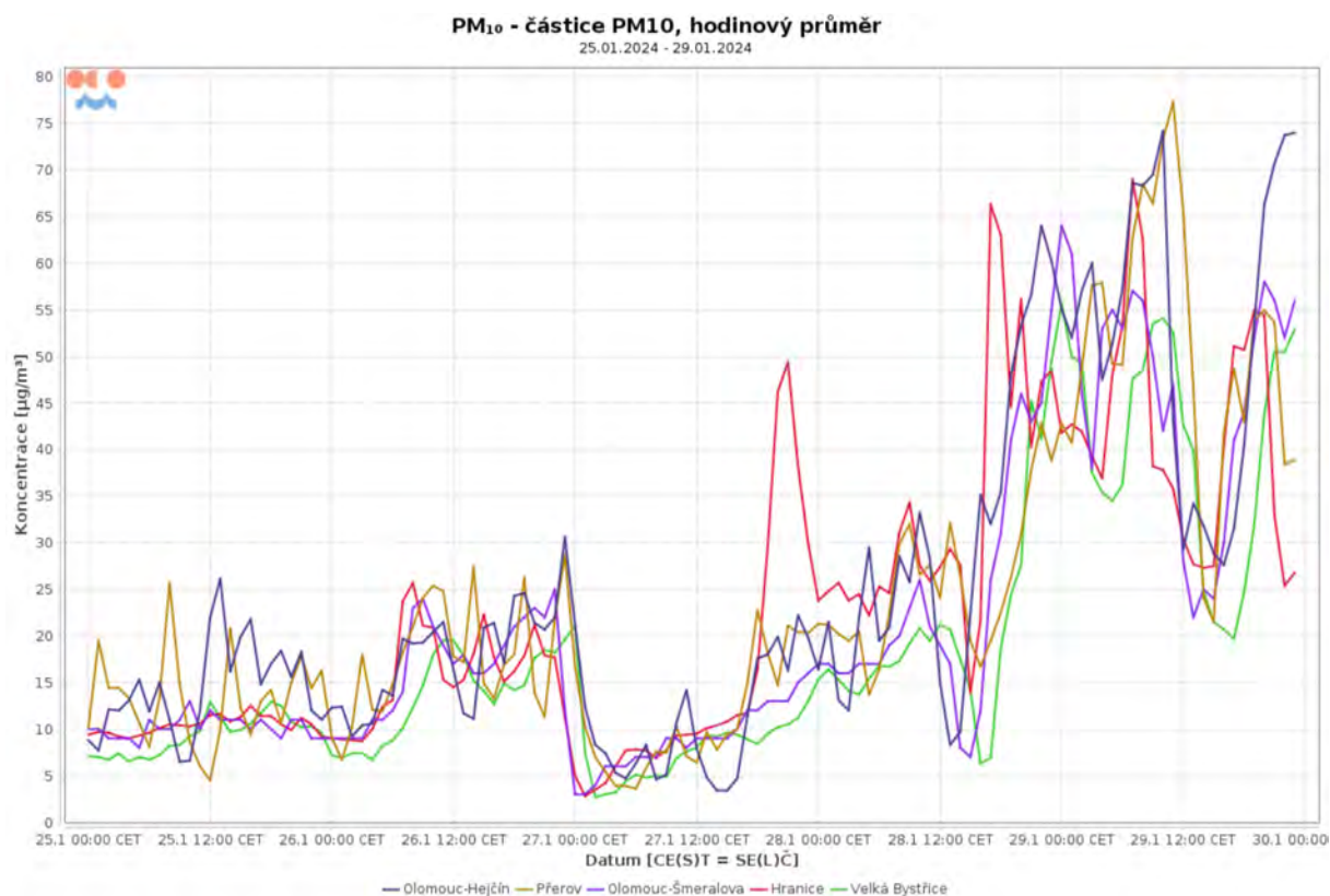
Obr. 5 Vzájemná korelace na stanicích ČHMÚ v Olomouckém kraji, hodinové koncentrace PM_{10} \mu\text{g}/\text{m}^3
