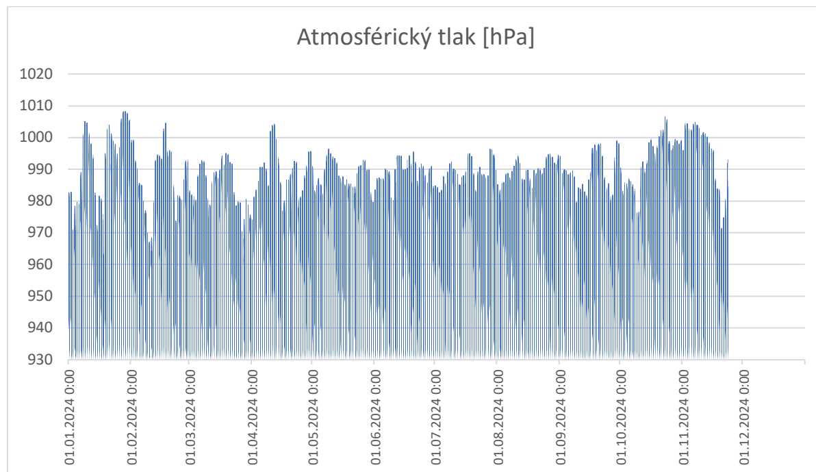
Obr. 17: Vývoj atmosférického tlaku na stanici 2524, včetně trendu.
