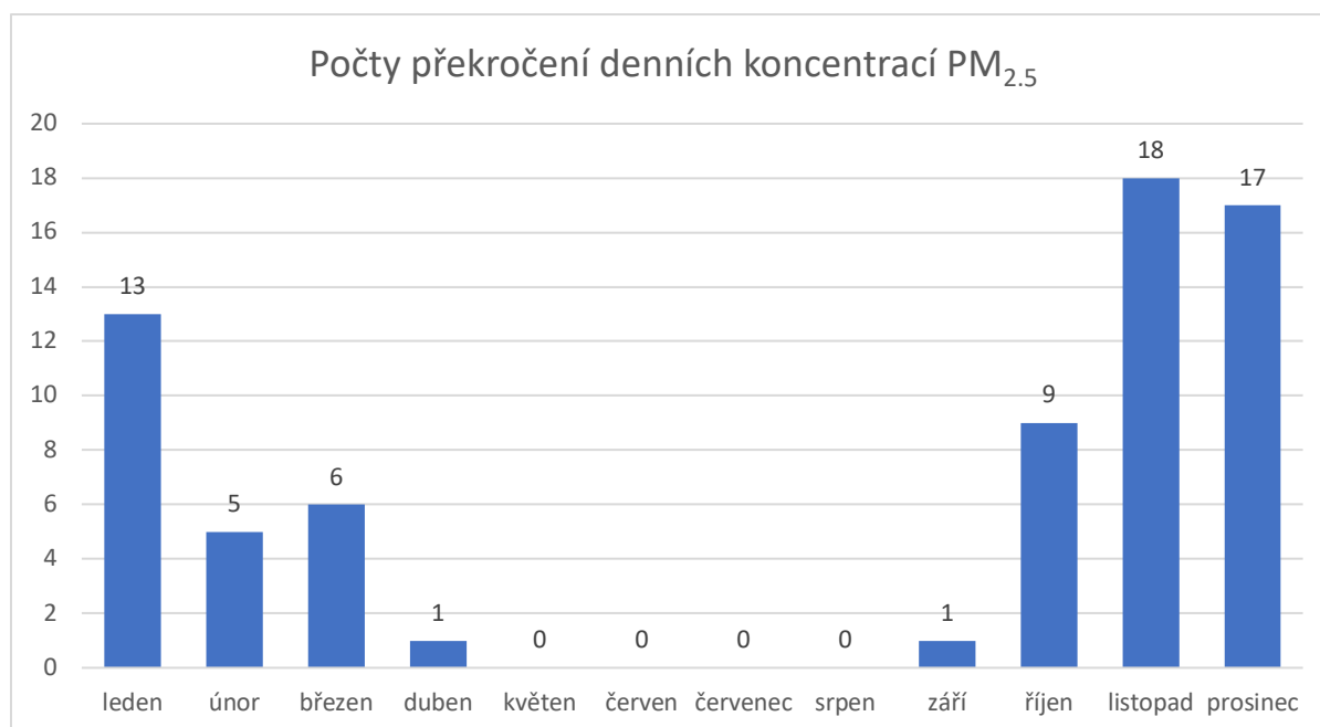
Obr.2: Četnost překročení DL v jednotlivých měsících na stanici 2524 pro PM 2.5
