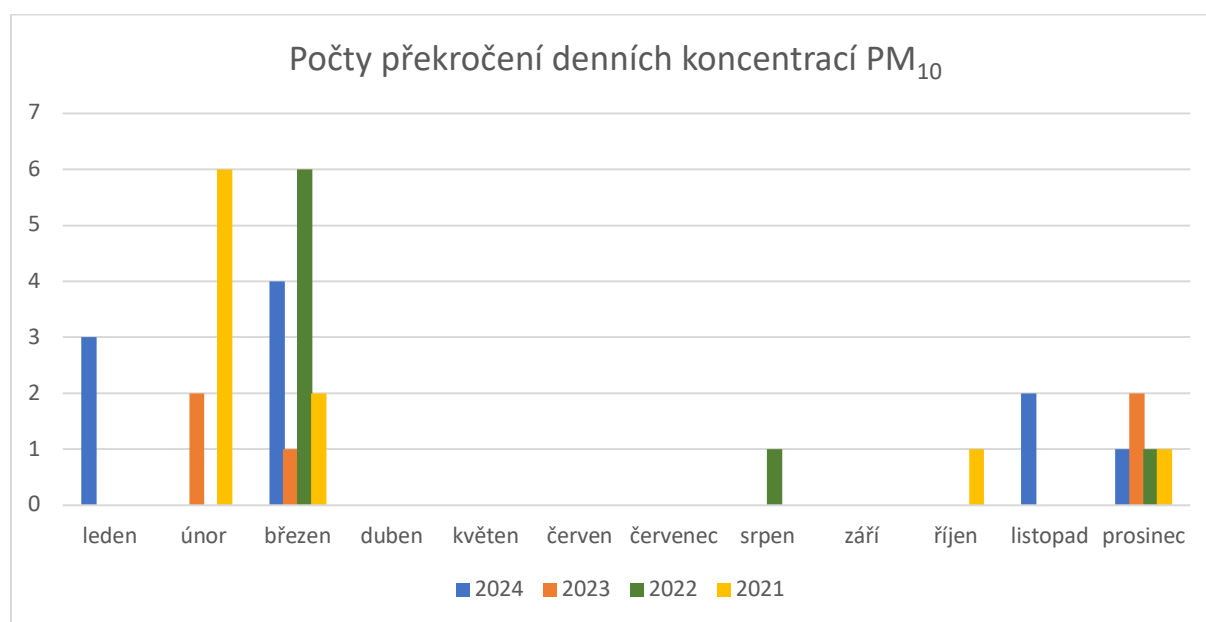
Obr.1: Četnost překročení DL v jednotlivých měsících na stanici 2524 pro PM 10
