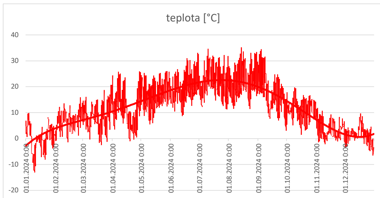
Obr. 15: Vývoj denních teplot na stanici 2524, včetně trendu.
