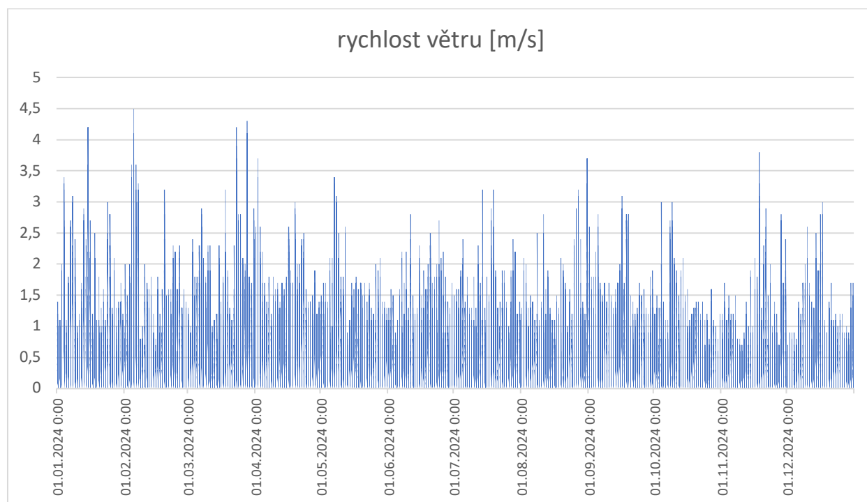
Obr. 12: Rychlost větru na stanici 2524 v hodinových údajích
