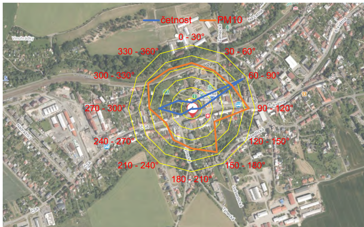
Obr. 14: Větrná růžice pro PM_{10} ve Velké Bystřici
