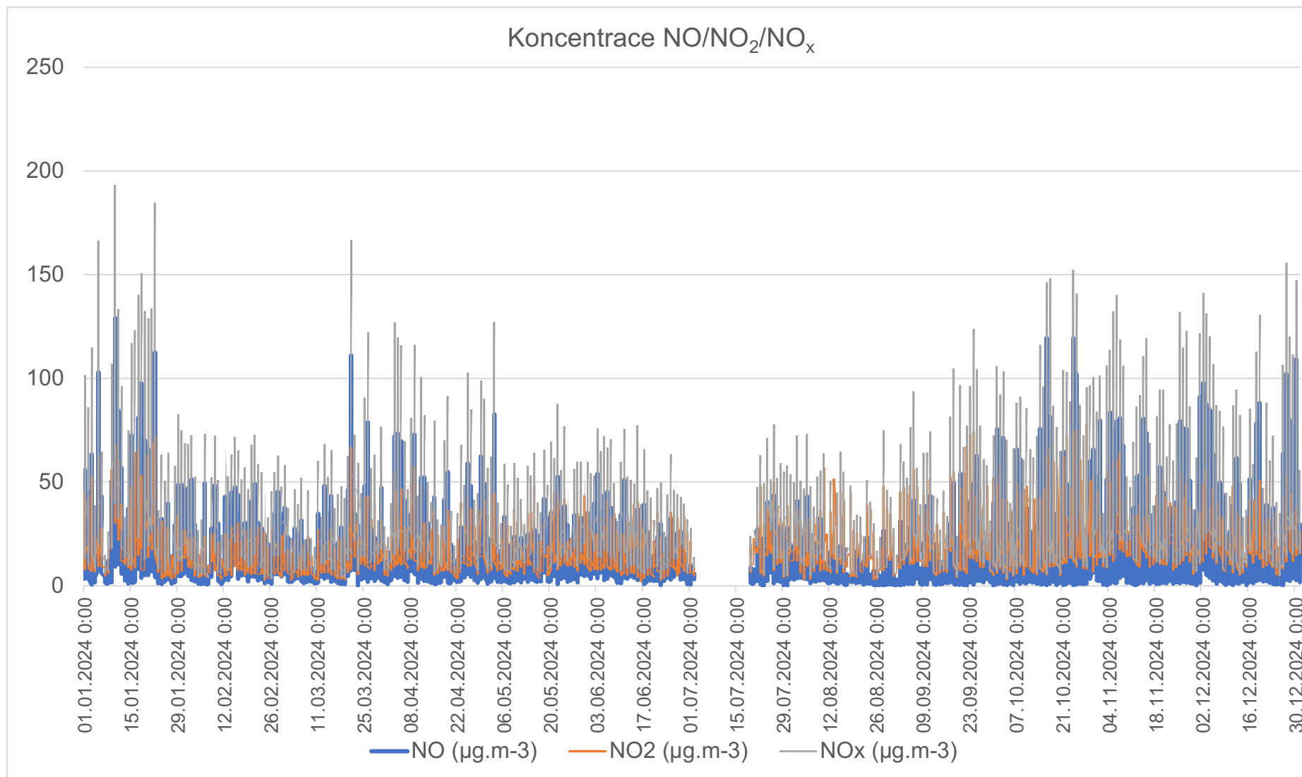
Obr. 8: Vývoj denních koncentrací NO x na stanici 2524, včetně trendu
