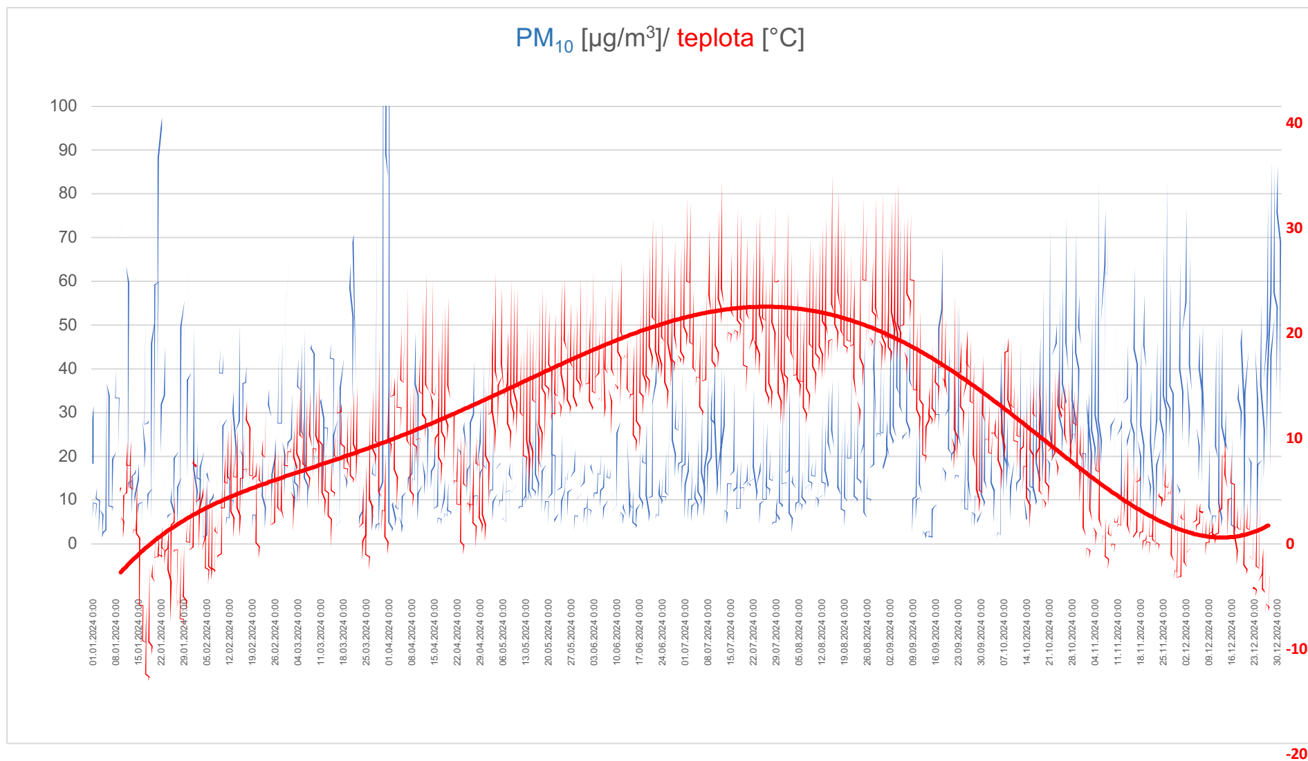
Obr. 4: Porovnání denních koncentrací PM 10 a teplot na stanici 2524.
