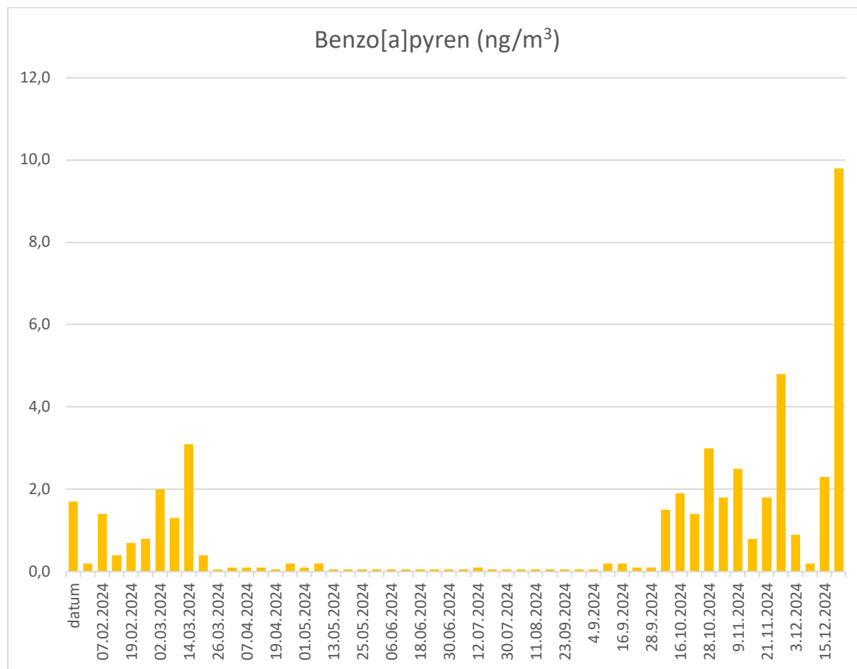
Obr. 11: Vývoj denních koncentrací benzo(a)pyrenu na stanici 2524.
