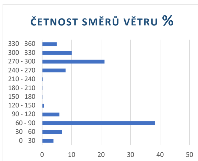
Obr. 13: Směrnost větru na stanici 2524 ve třídách po 30°.
