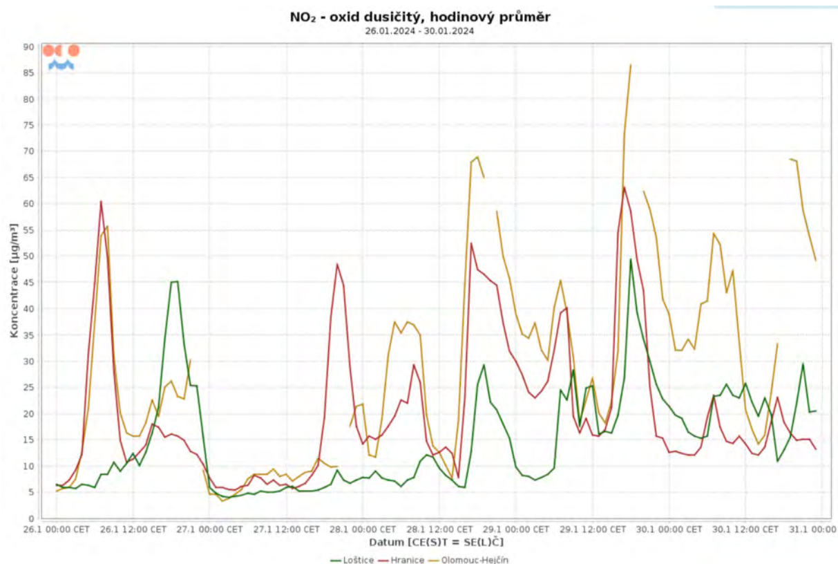
Obr. 10: Vzájemná korelace na stanicích ČHMÚ v Olomouckém kraji, hodinové koncentrace NO 2 µg/m 3
