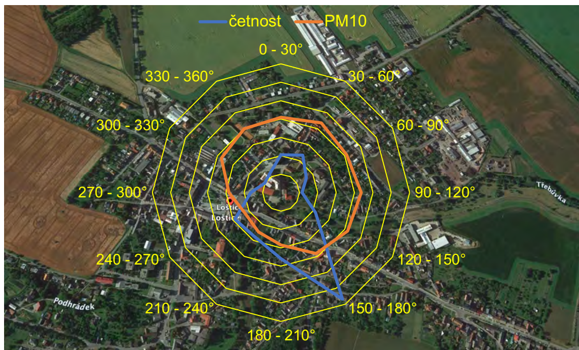
Obr. 14: Větrná růžice pro PM_{10} v Lošticích
