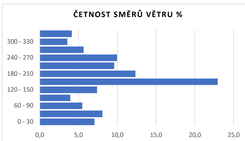
Obr. 13: Směrnost větru na stanici 2299 ve třídách po 30°.
