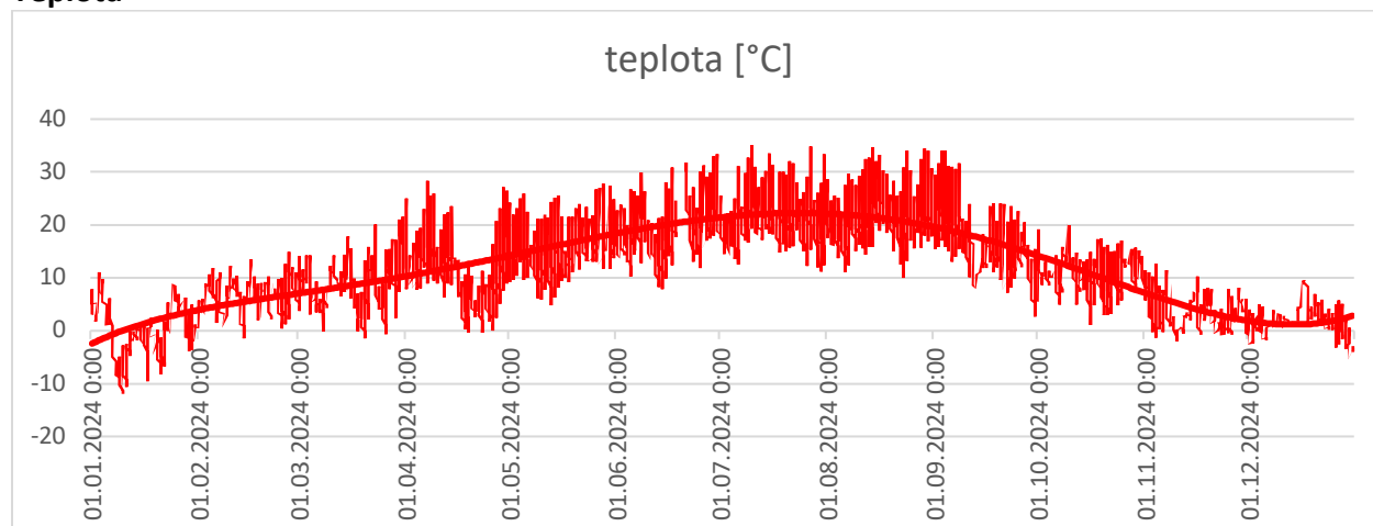
Obr. 15: Vývoj denních teplot na stanici 2299, včetně trendu.
