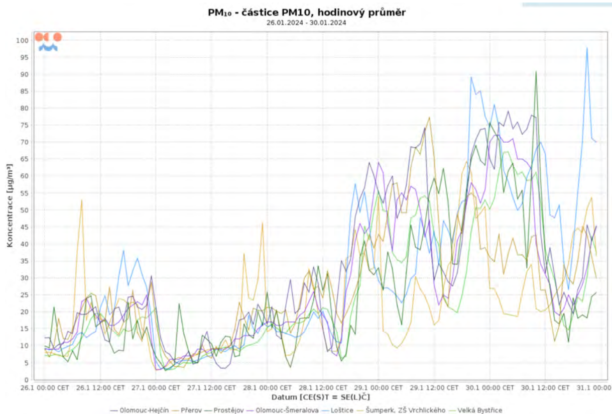
Obr. 5 Vzájemná korelace na stanicích ČHMÚ v Olomouckém kraji, hodinové koncentrace PM_{10} µg/m 3
