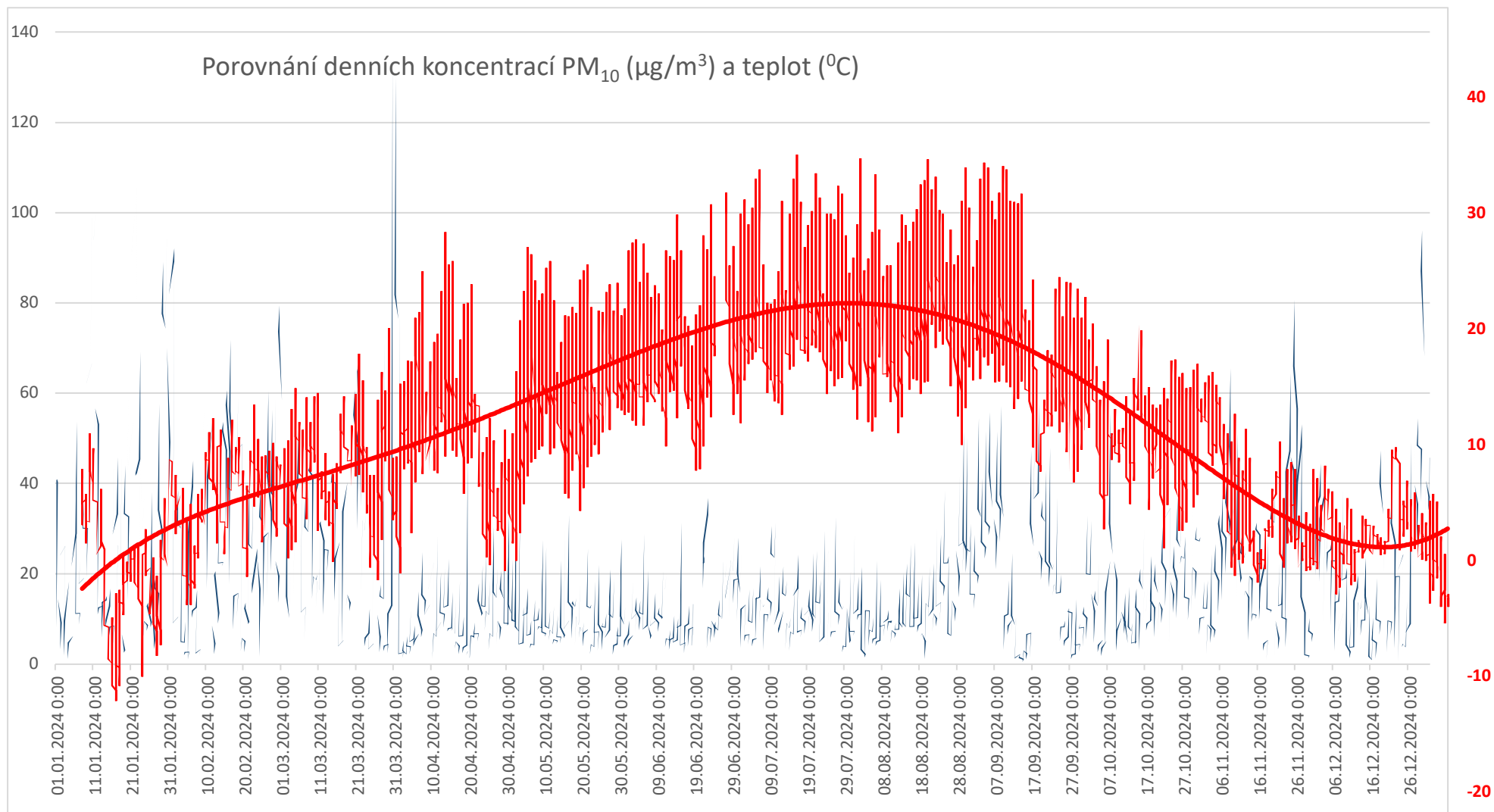
Obr. 4: Porovnání denních koncentrací PM 10 a teplot podle sezón na stanici 2299.
