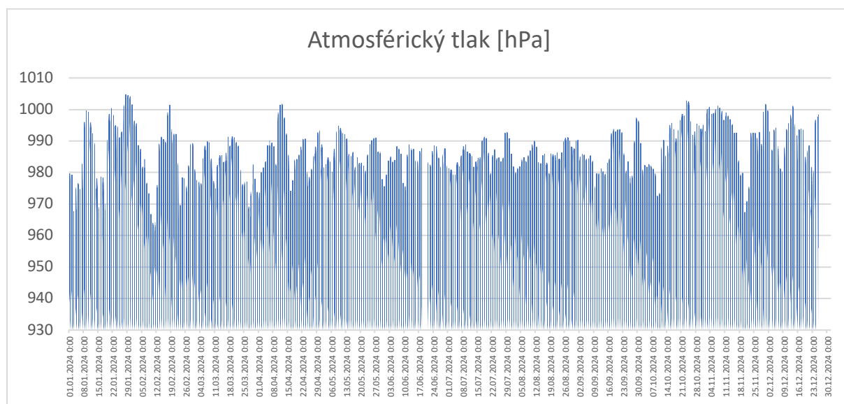
Obr. 17: Vývoj atmosférického tlaku na stanici 2299, včetně trendu.
