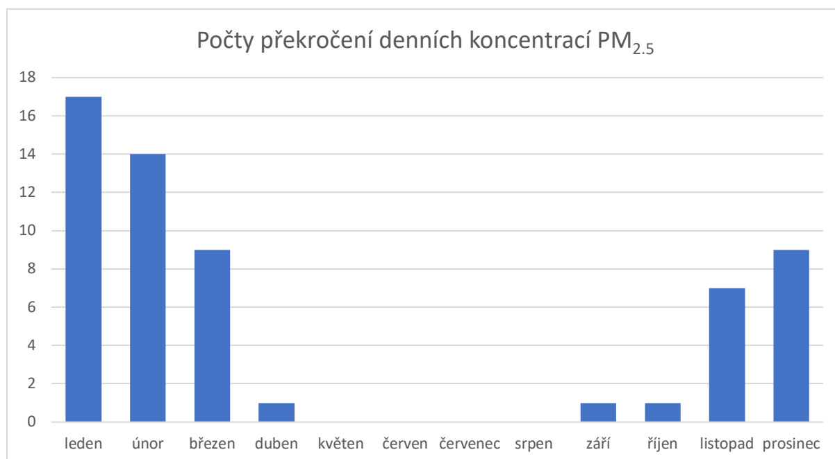
Obr.2: Četnost překročení DL v jednotlivých měsících na stanici 2299 pro PM 2.5
