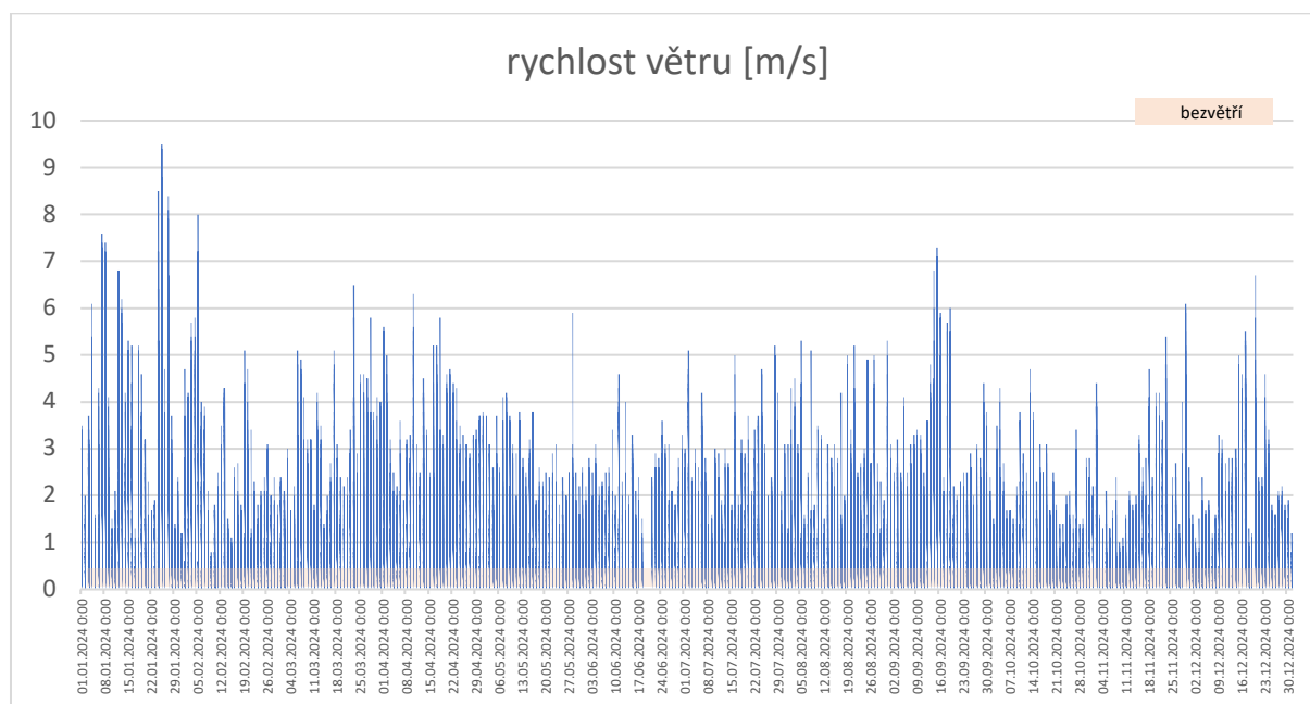
Obr. 12: Rychlost větru na stanici 2299 v hodinových údajích
