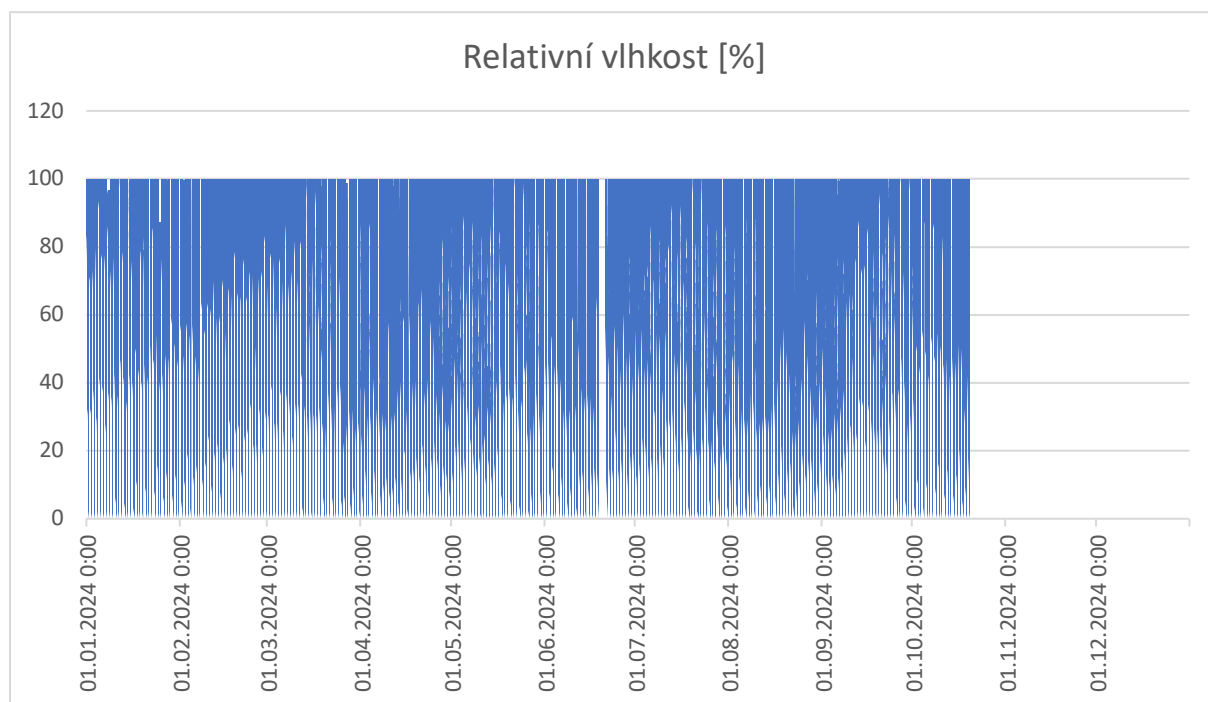
Obr. 16: Vývoj relativní vlhkosti na stanici 2299, včetně trendu.
