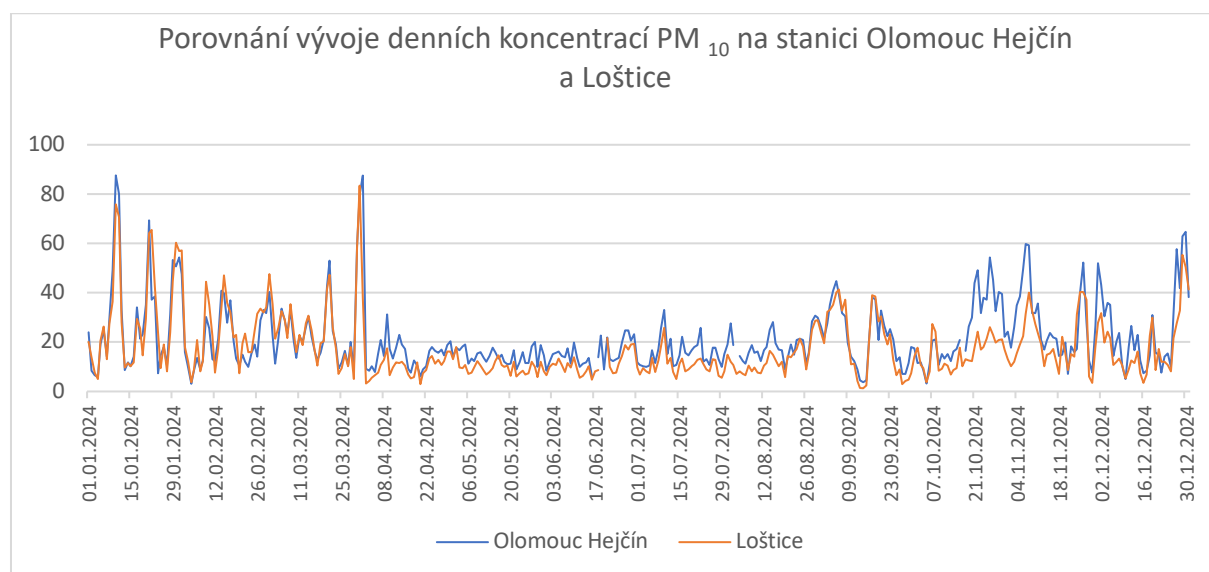
Obr.7: Souběh denních koncentrací PM 10 na porovnávaných stanicích
