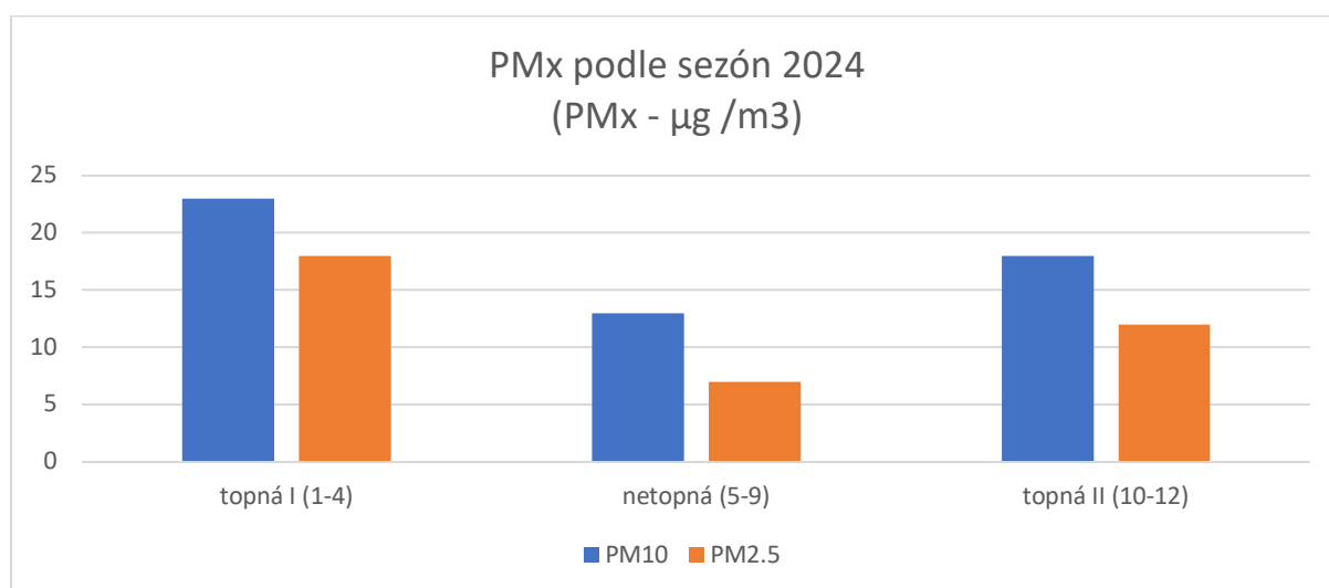
Obr. 3: Porovnání průměrných hodnot PM x podle sezón na stanici 2299 pro rok 2024
