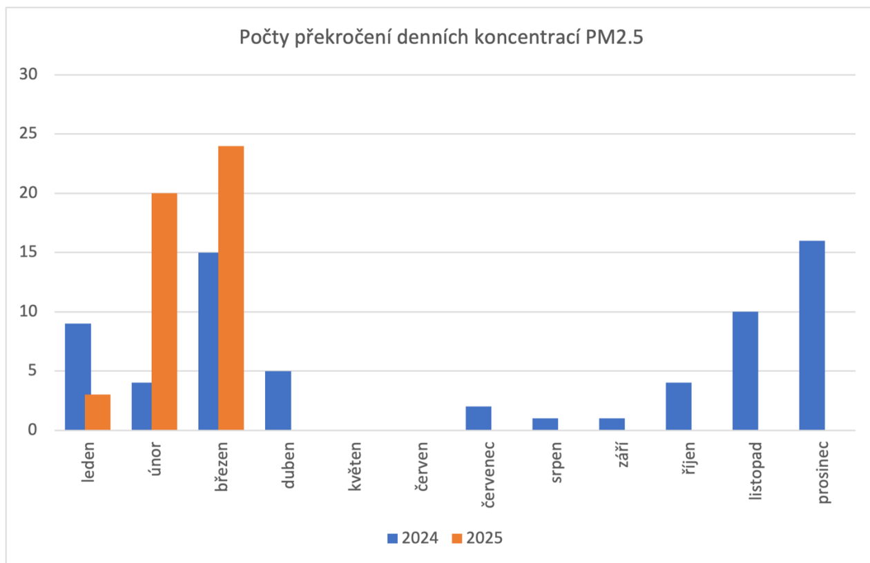
Obr.2: Četnost překročení DL v jednotlivých měsících na stanici 2293 pro PM 2.5
