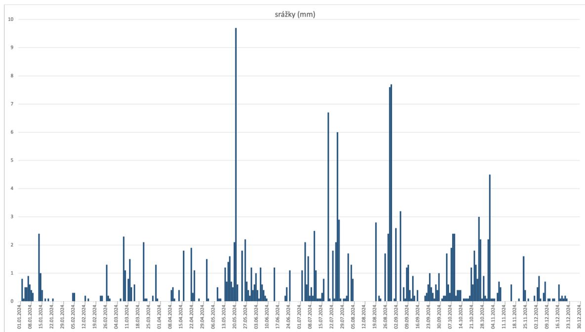
Obr. 15: Vývoj denních úhrnů srážek (mm) na stanici 2293, včetně trendu.
