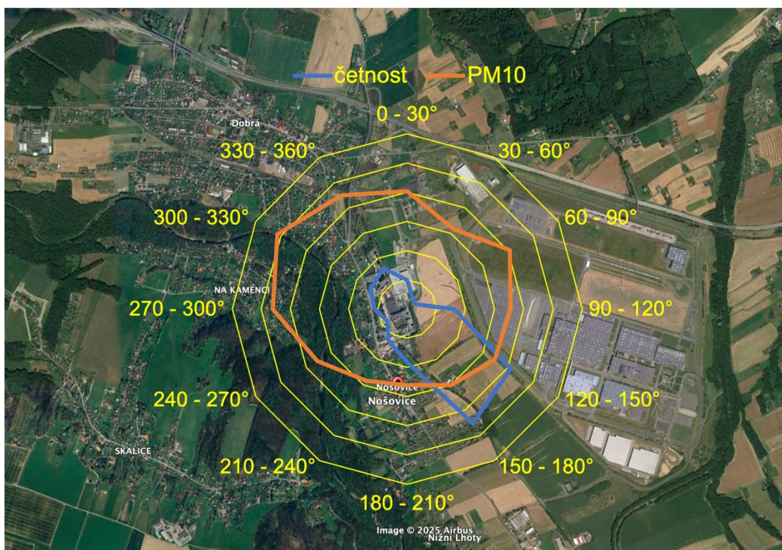
Obr. 12: Směrnost větru na stanici 2293 ve třídách po 30°. Rozdělení směrnosti větrů jasně prokázalo dominantní směry 150–210 stupňů, stejně jako v předchozích letech. Převládá tedy jižní až jihozápadní vítr. Nejméně se vyskytuje vítr východní.
