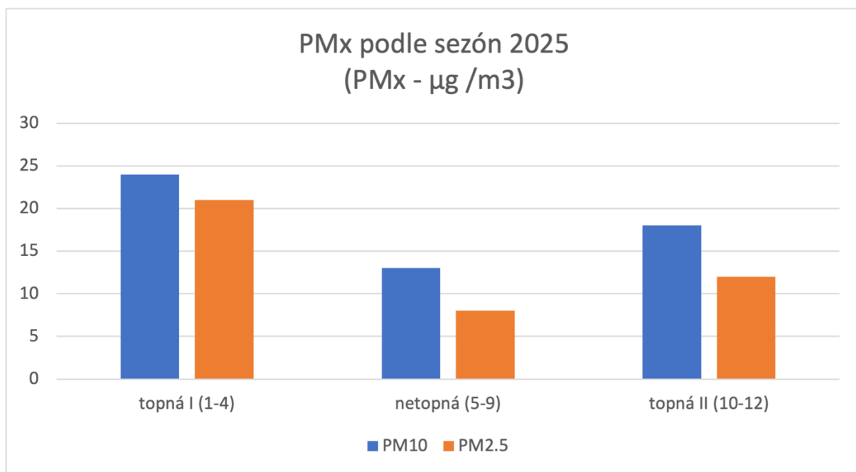
Obr. 3: Porovnání průměrných hodnot PM x podle sezón na stanici 2293.
