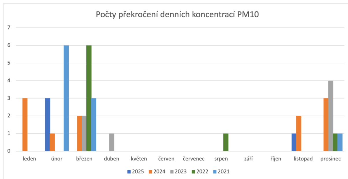
Obr. 1: Počty překročení denních koncentrací, překračujících DL pro PM10 na stanici 2293.
