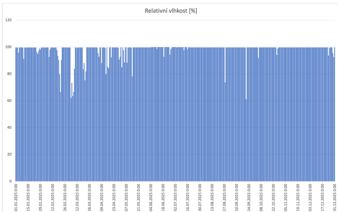
Obr. 16: Vývoj relativní vlhkosti na stanici 2293, včetně trendu.
