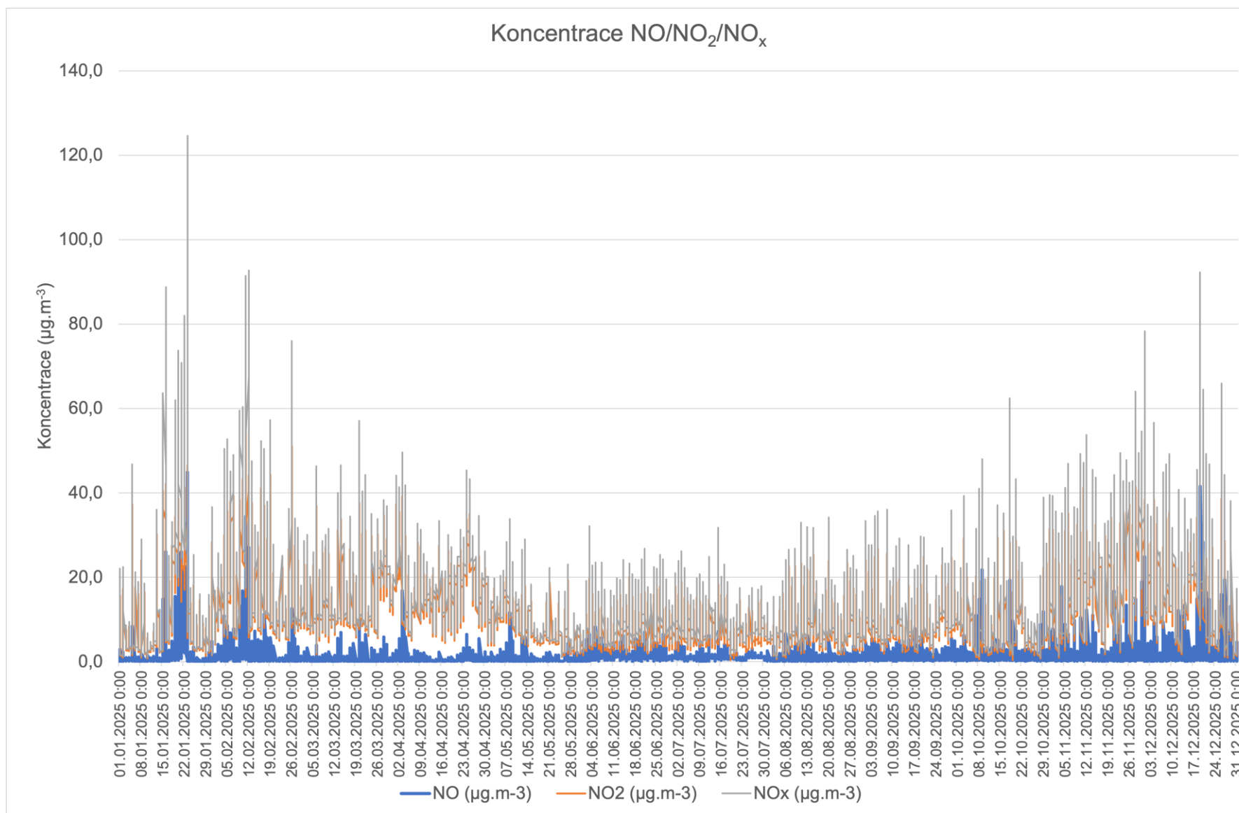
Obr. 8: Vývoj denních koncentrací NO x na stanici 2293, včetně trendu.
