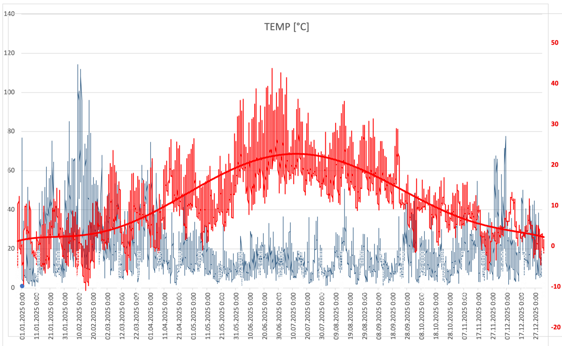
Obr. 4: Porovnání denních koncentrací PM 10 a teplot podle sezón na stanici 2293.
