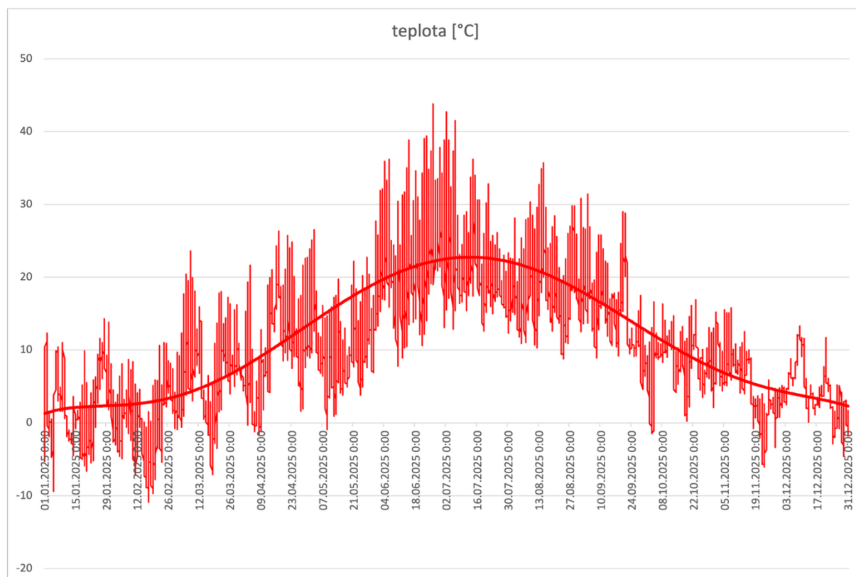
Obr. 14: Vývoj denních teplot na stanici 2293
