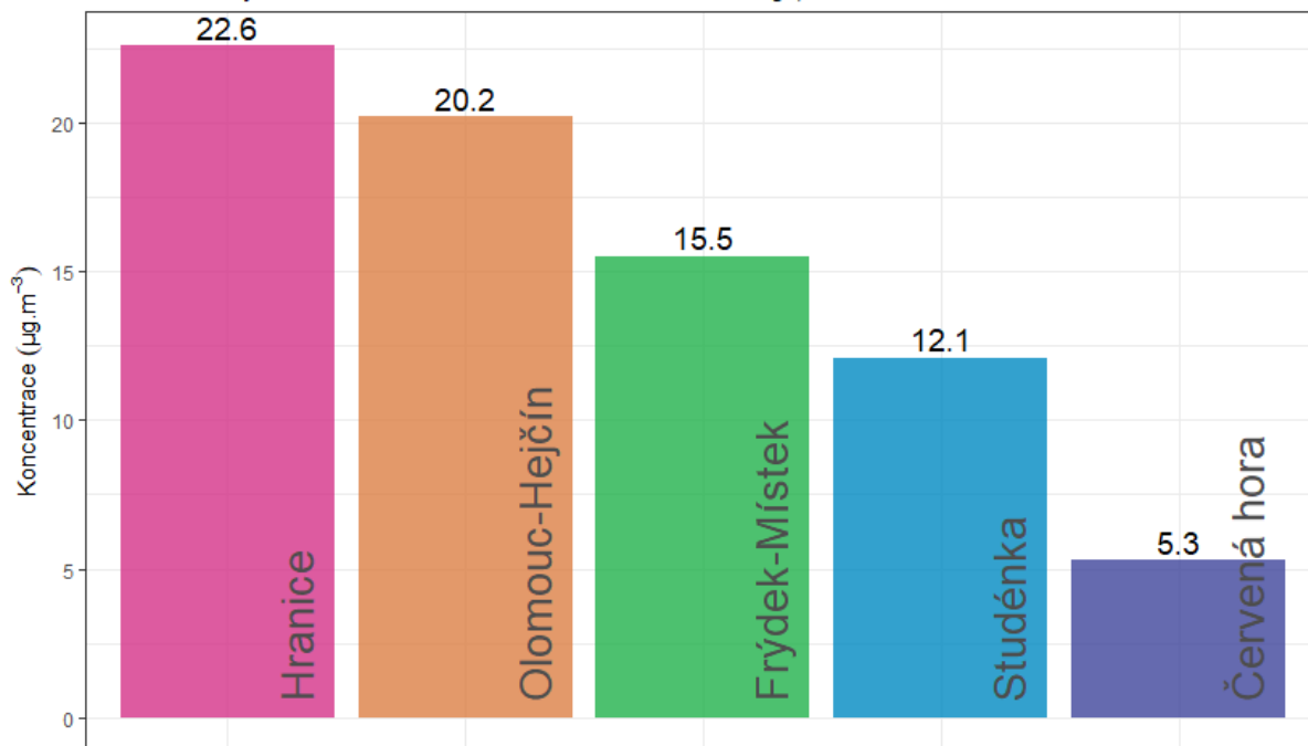
Obr. 52 – Srovnání průměrné roční koncentrace NO 2 lokality Hranice s okolními stanicemi státní sítě imisního monitoringu, rok 2019
