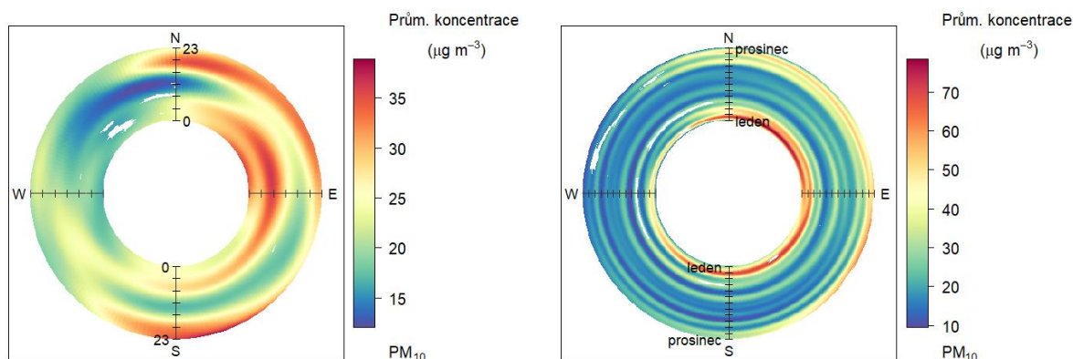
Obr. 31 – Průměrný denní chod (vlevo) a roční chod (vpravo) koncentrací dle směru větru, Hranice, rok 2019
