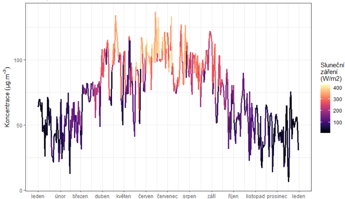
Obr. 59 – Vliv slunečního záření na koncentrace O 3 , Hranice, rok 2019
