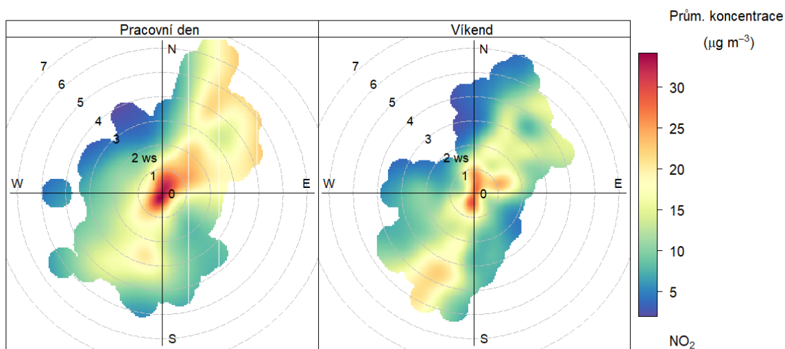
Obr. 48 – Koncentrační růžice NO 2 v pracovní dny a o víkendu, lokalita Hranice, rok 2019
