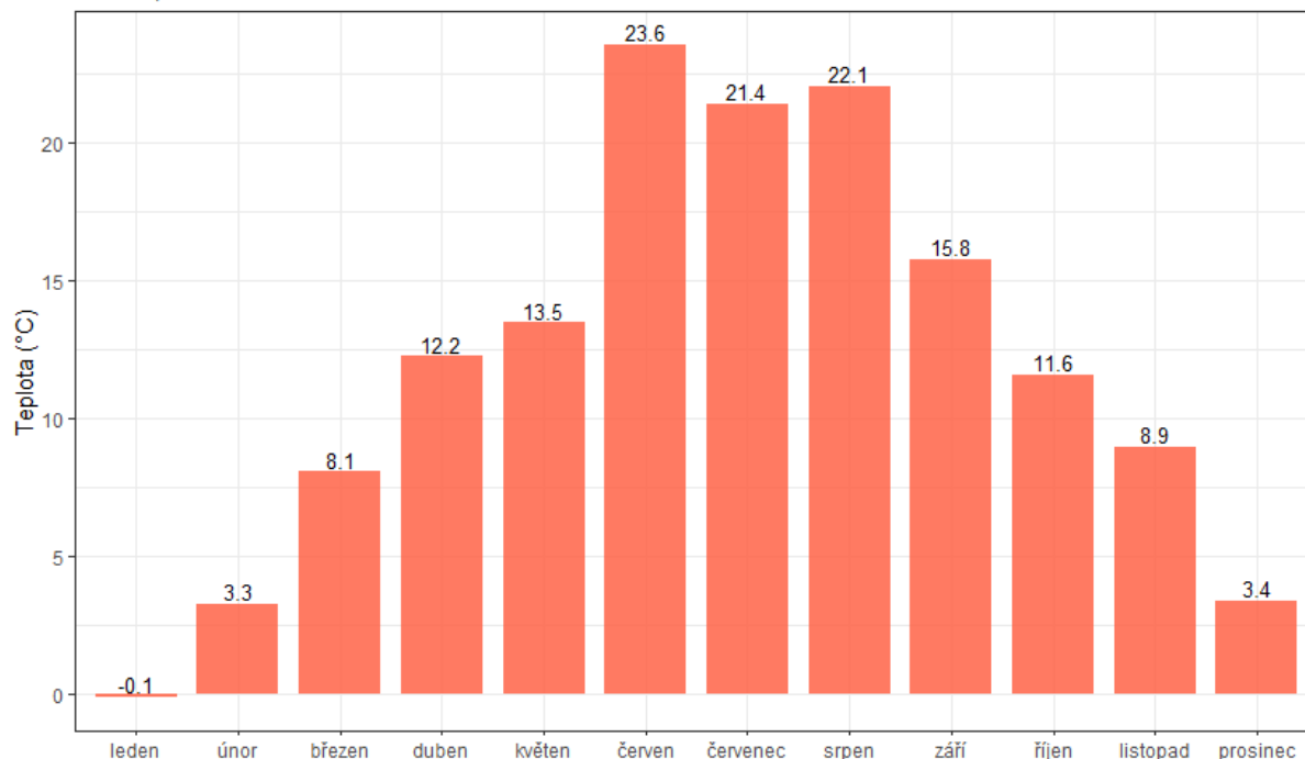
Obr. 5 – Průměrné měsíční teploty, Hranice, rok 2019
