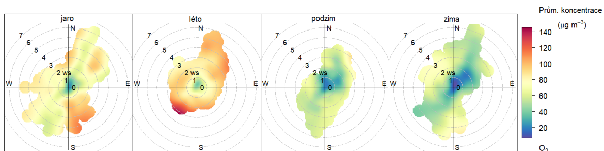
Obr. 64 – Koncentrační růžice jednotlivých ročních období, Hranice, rok 2019
