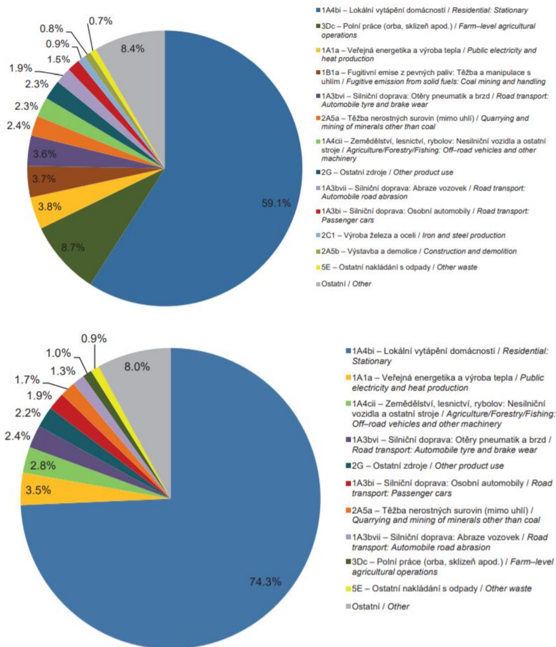
Obr. 15 – Podíl sektorů NFR na celkových emisích PM 10 (nahore) a PM 2,5 (dole) v ČR, rok 2017 [5]
