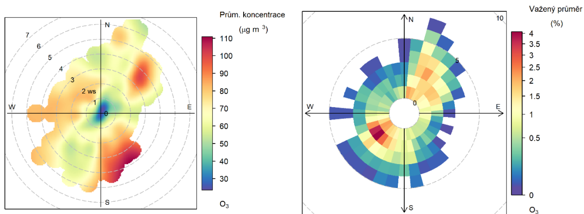
Obr. 62 – Koncentrační růžice (vlevo) a vážená koncentrační růžice (vpravo) pro O 3 , Hranice, rok 2019
