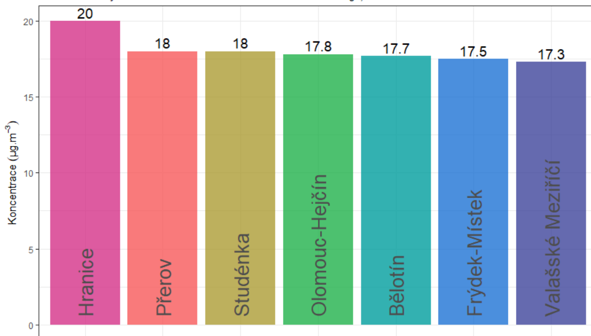
Obr. 33 – Srovnání průměrné roční koncentrace PM 2,5 lokality Hranice s okolními stanicemi státní sítě imisního monitoringu, rok 2019
