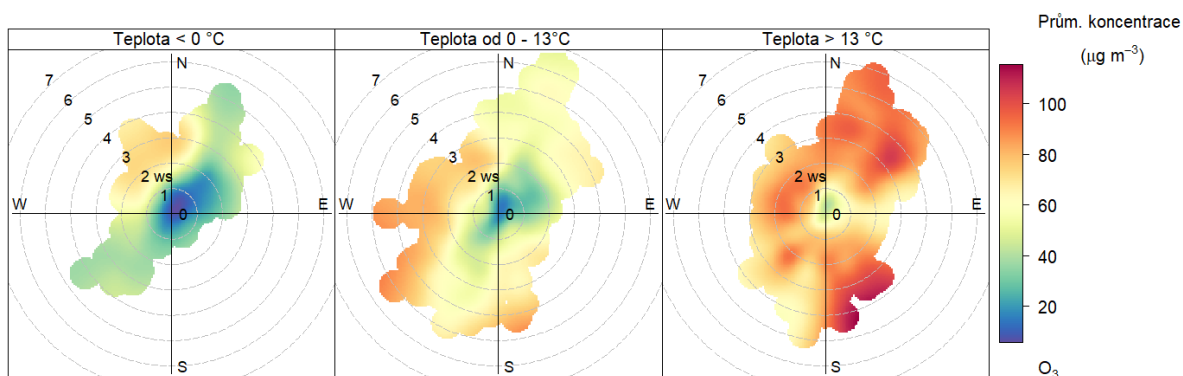
Obr. 65 – Koncentrační růžice členěná dle teplot, Hranice, rok 2019
