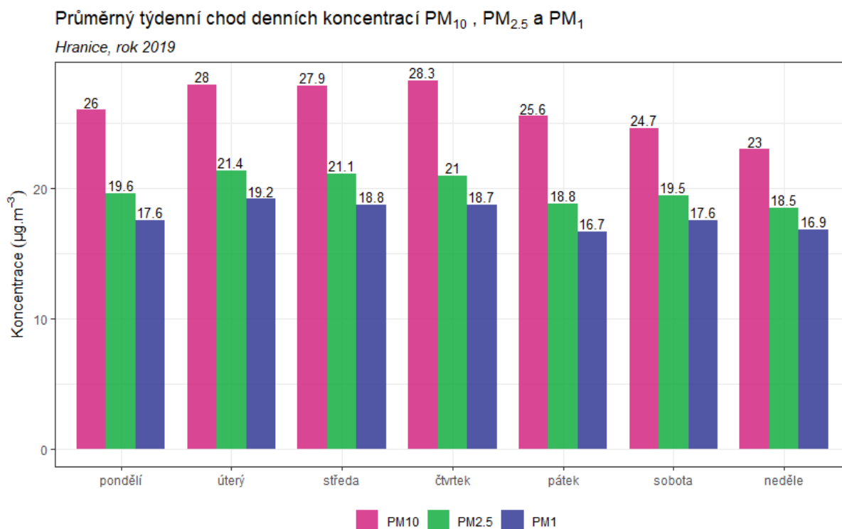
Obr. 25 – Průměrný týdenní chod denních koncentrací PM 10 , Hranice, rok 2019
