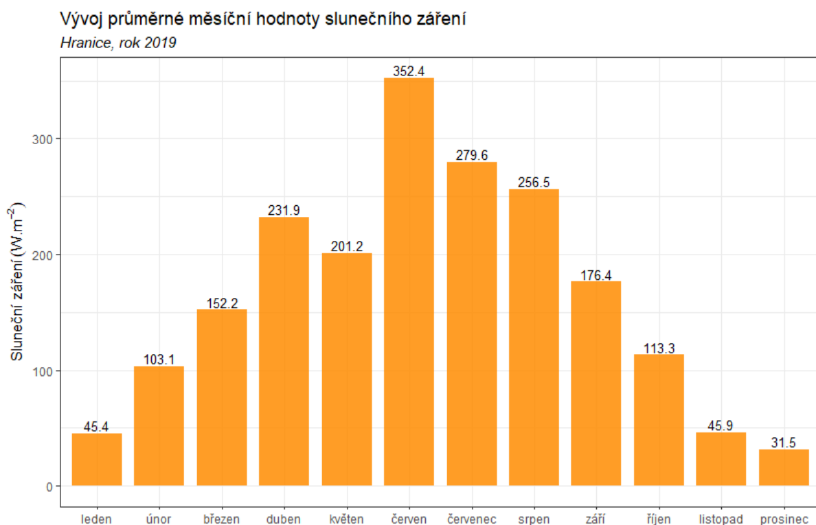
Obr. 11 – Průměrné měsíční hodnoty slunečního záření, Hranice, rok 2019
