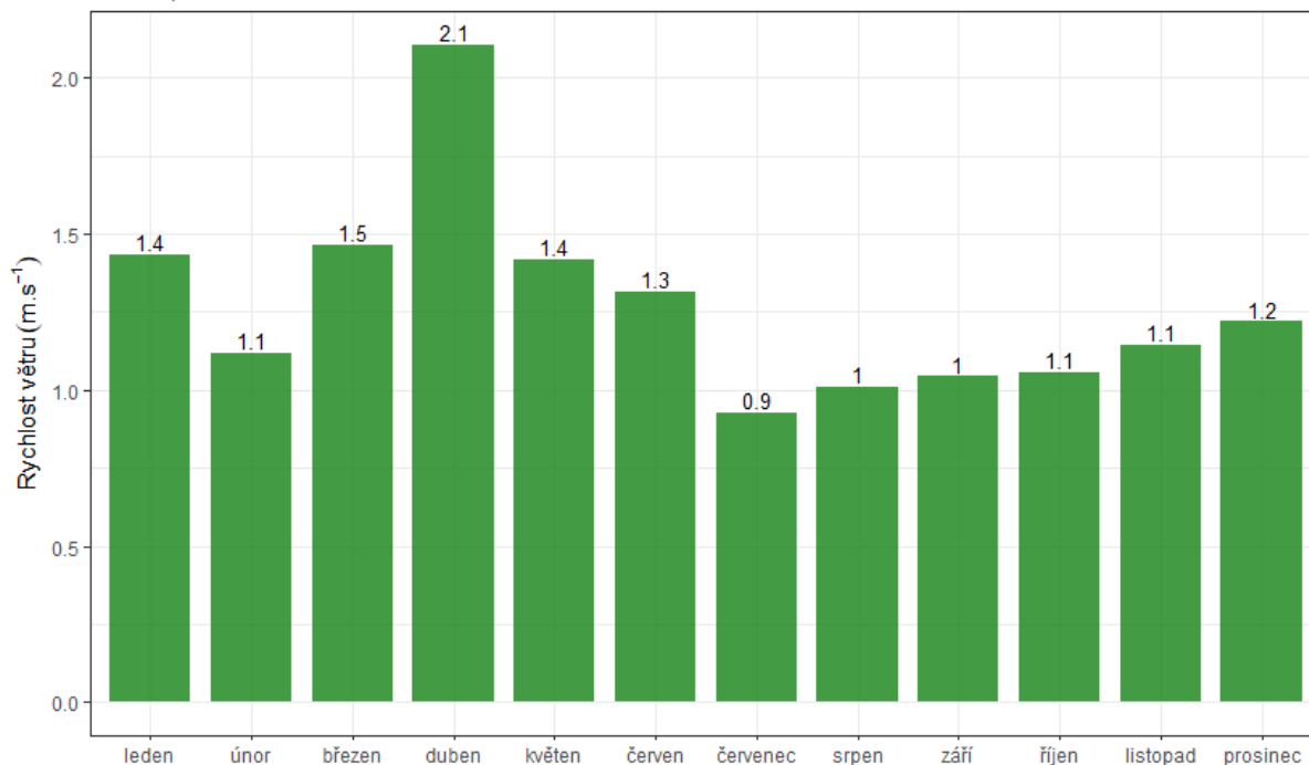
Obr. 3 – Průměrné měsíční rychlosti větru, Hranice, rok 2019
