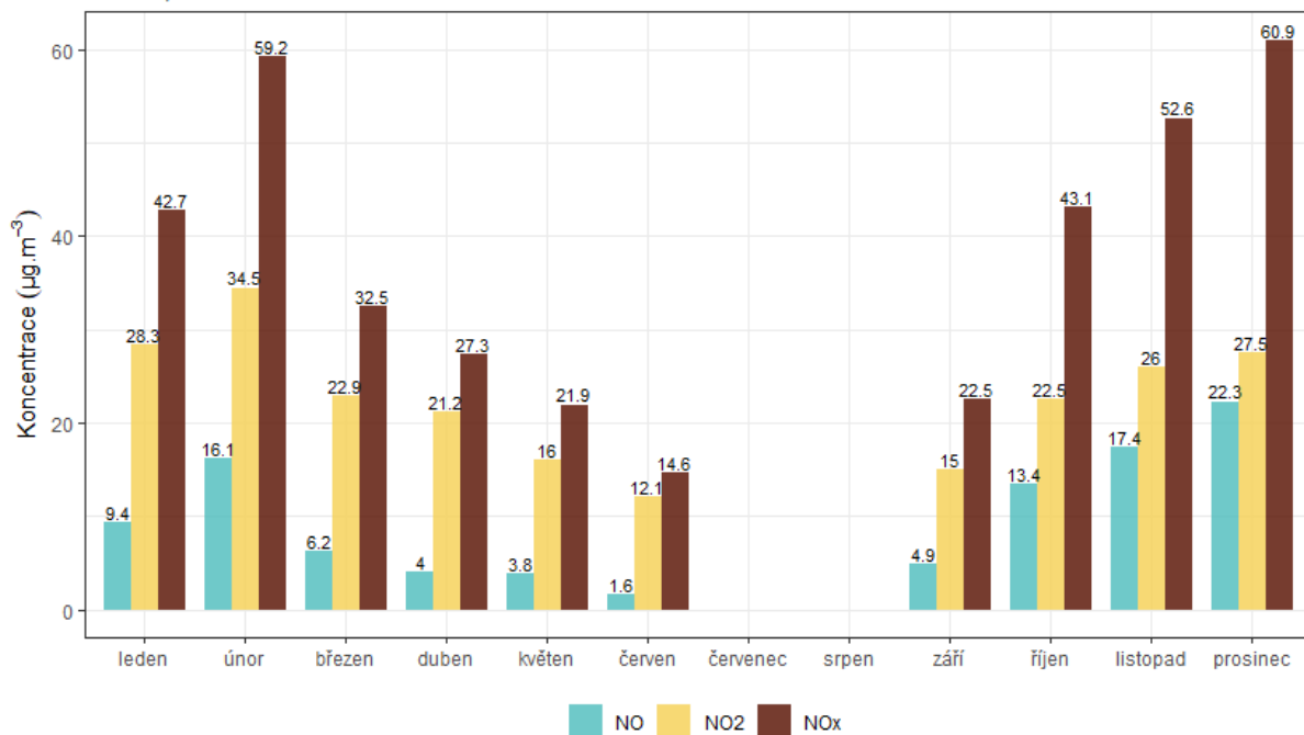
Obr. 40 - Průměrné měsíční koncentrace NO, NO 2 a NO x , Hranice, rok 2019
