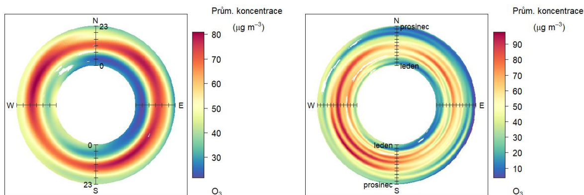
Obr. 66 – Průměrný denní chod (vlevo) a roční chod (vpravo) koncentrací dle směru větru, Hranice, rok 2019
