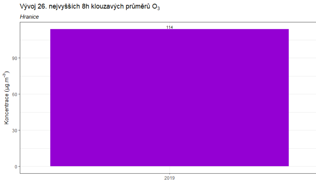
Obr. 54 – Vývoj 26. nejvyššího 8hodinového klouzavého průměru O 3 za den, lokalita Hranice
