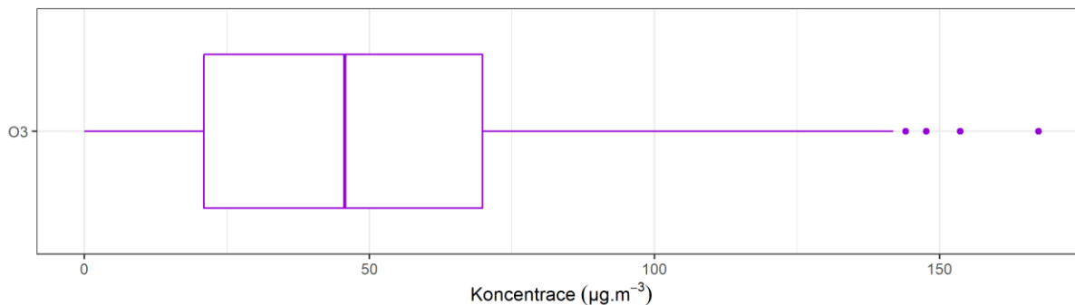
Obr. 55 – Statistické zpracování hodinových koncentrací O 3 v lokalitě Hranice, rok 2019
