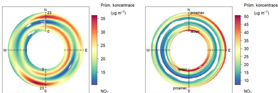
Obr. 51 – Průměrný denní chod (vlevo) a roční chod (vpravo) koncentrací dle směru větru, Hranice, rok 2019
