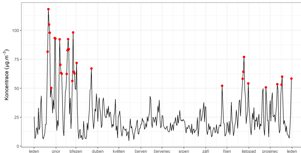
Obr. 23 – Výskyt dní s překročenou hodnotou denního imisního limitu pro PM 10 , lokalita Hranice, rok 2019
