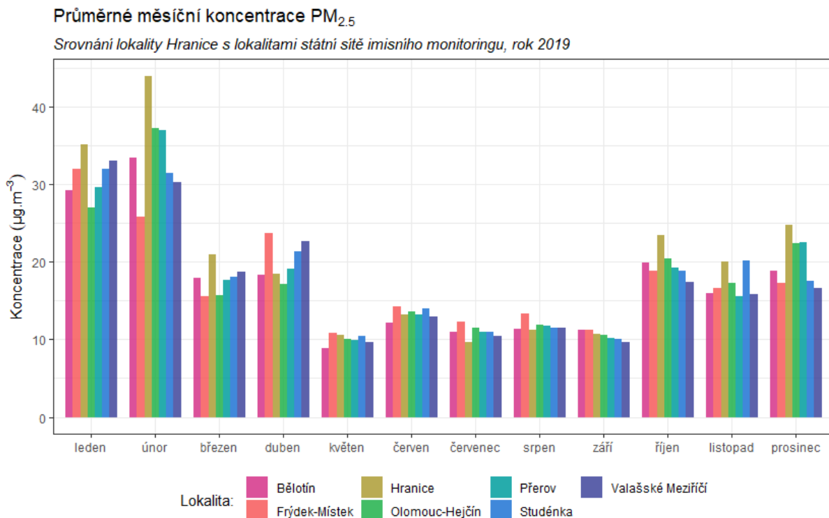
Obr. 36 – Srovnání průměrných měsíčních koncentrací PM 2,5 lokality Hranice s okolními stanicemi státní sítě imisního monitoringu, rok 2019
