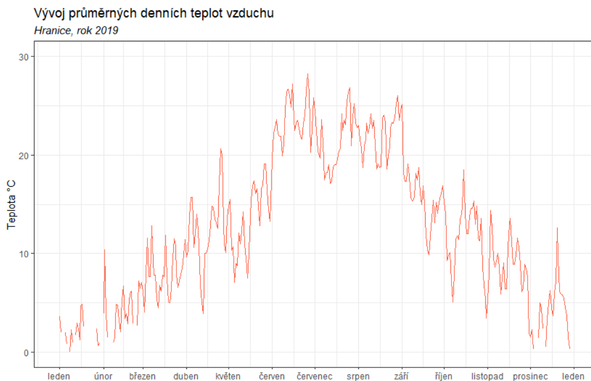
Obr. 4 – Průměrné denní teploty vzduchu, Hranice, rok 2019
