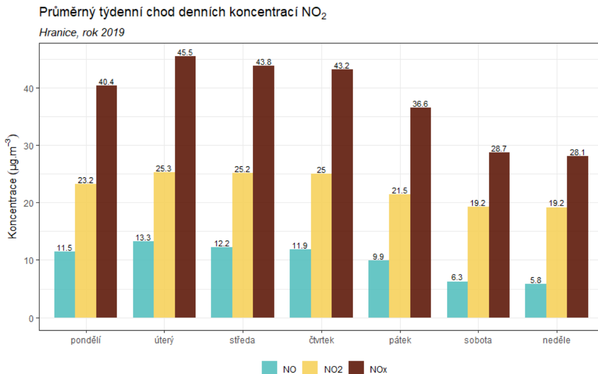
Obr. 44 – Průměrný týdenní chod denních koncentrací NO 2 , Hranice, rok 2019
