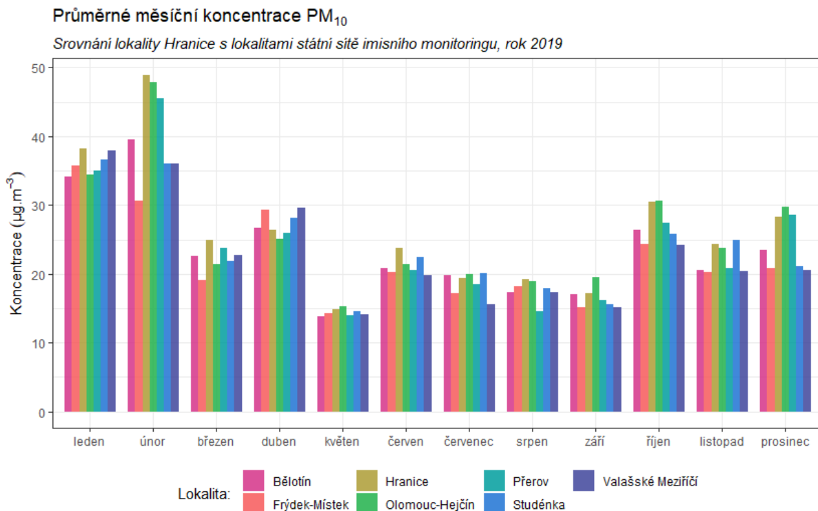
Obr. 35 – Srovnání průměrných měsíčních koncentrací PM 10 lokality Hranice s okolními stanicemi státní sítě imisního monitoringu, rok 2019
