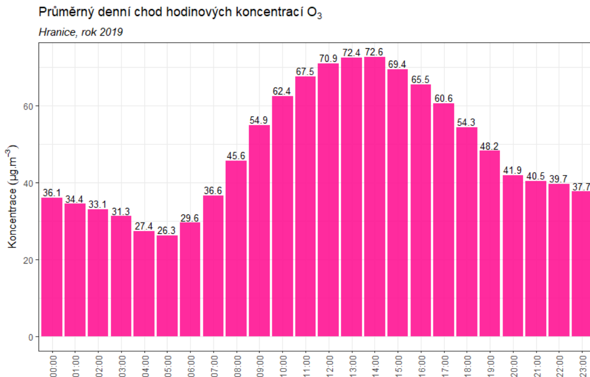
Obr. 61 – Denní chod hodinových koncentrací O_3 , Hranice, rok 2019
