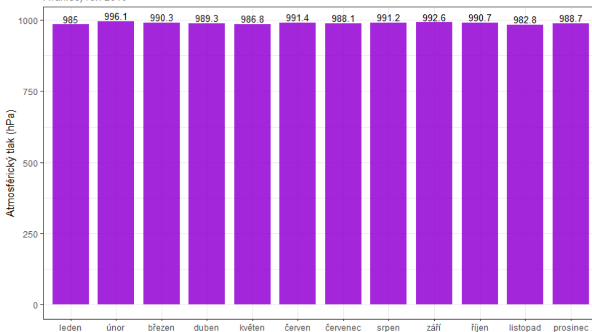
Obr. 13 – Průměrné měsíční hodnoty atmosférického tlaku, Hranice, rok 2019
