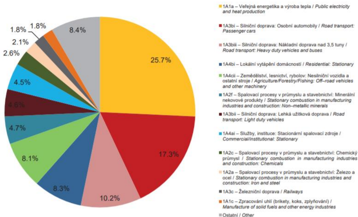
Obr. 37 – Podíl sektorů NFR na celkových emisích NO x v ČR, rok 2017 [5]
