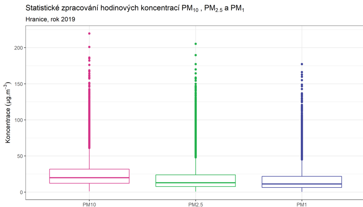
Obr. 17 – Statistické zpracování hodinových koncentrací PM 10 , PM 2,5 a PM 1 v lokalitě Hranice, rok 2019
