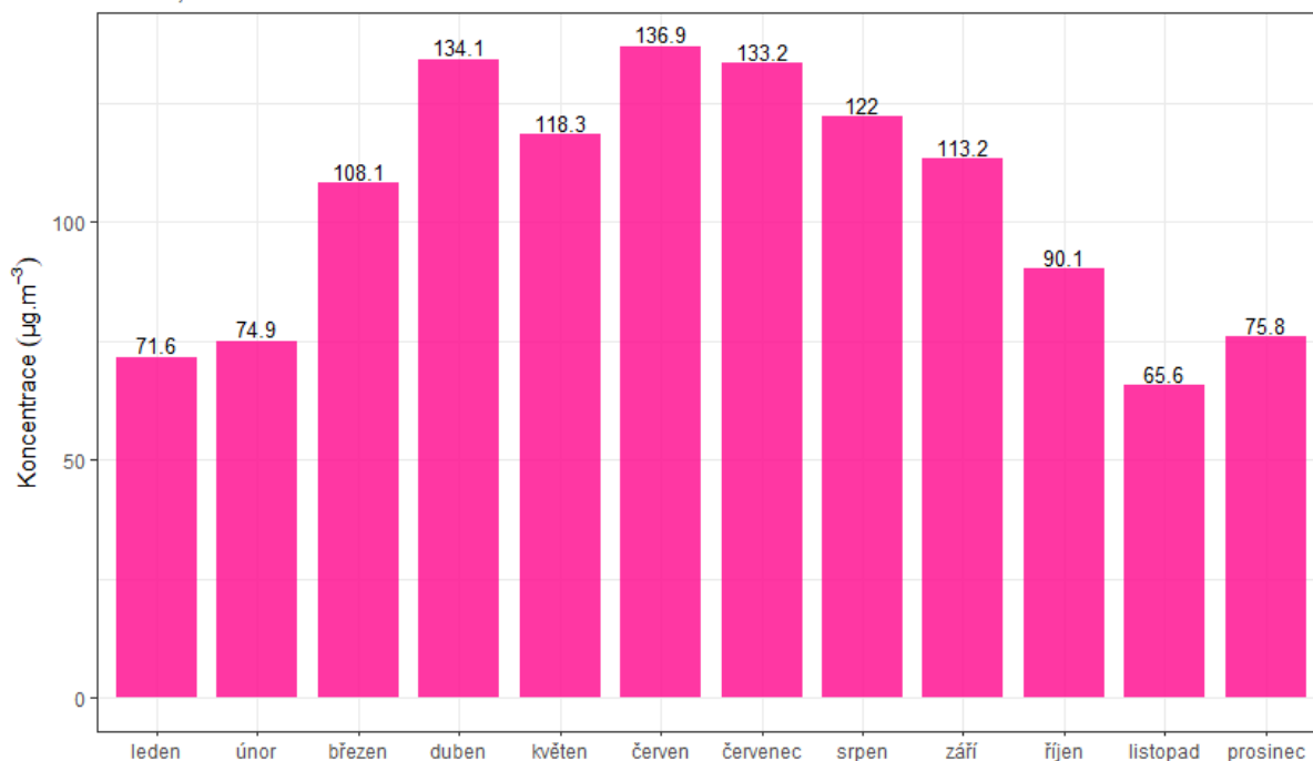
Obr. 56 – Maximální 8h klouzavé průměry O_3 za den v jednotlivých měsících, Hranice, rok 2019
