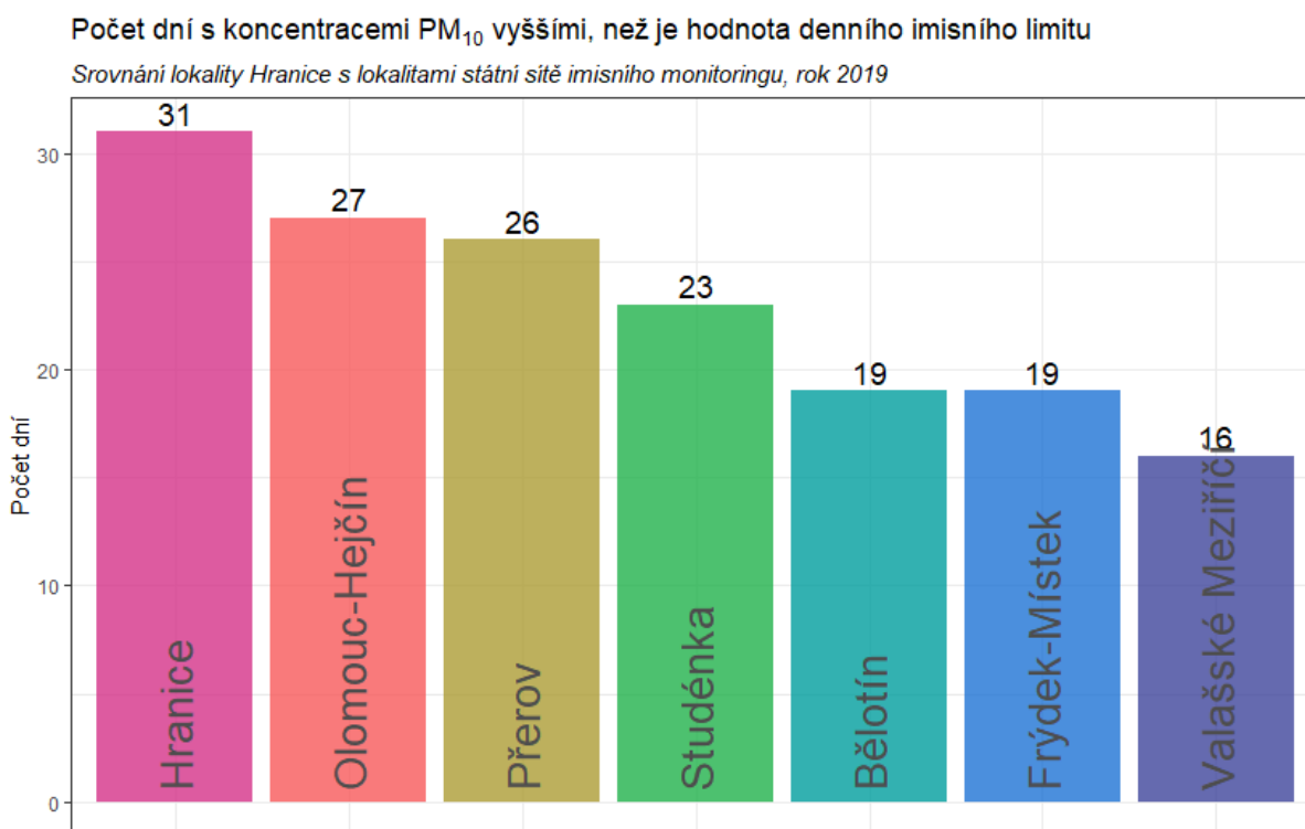
Obr. 34 – Počet dní s průměrnými denními koncentracemi PM_{10} vyššími, než je hodnota imisního limitu pro průměrnou denní koncentraci PM_{10} , srovnání lokality Hranice s okolními stanicemi státní sítě imisního monitoringu, rok 2019
