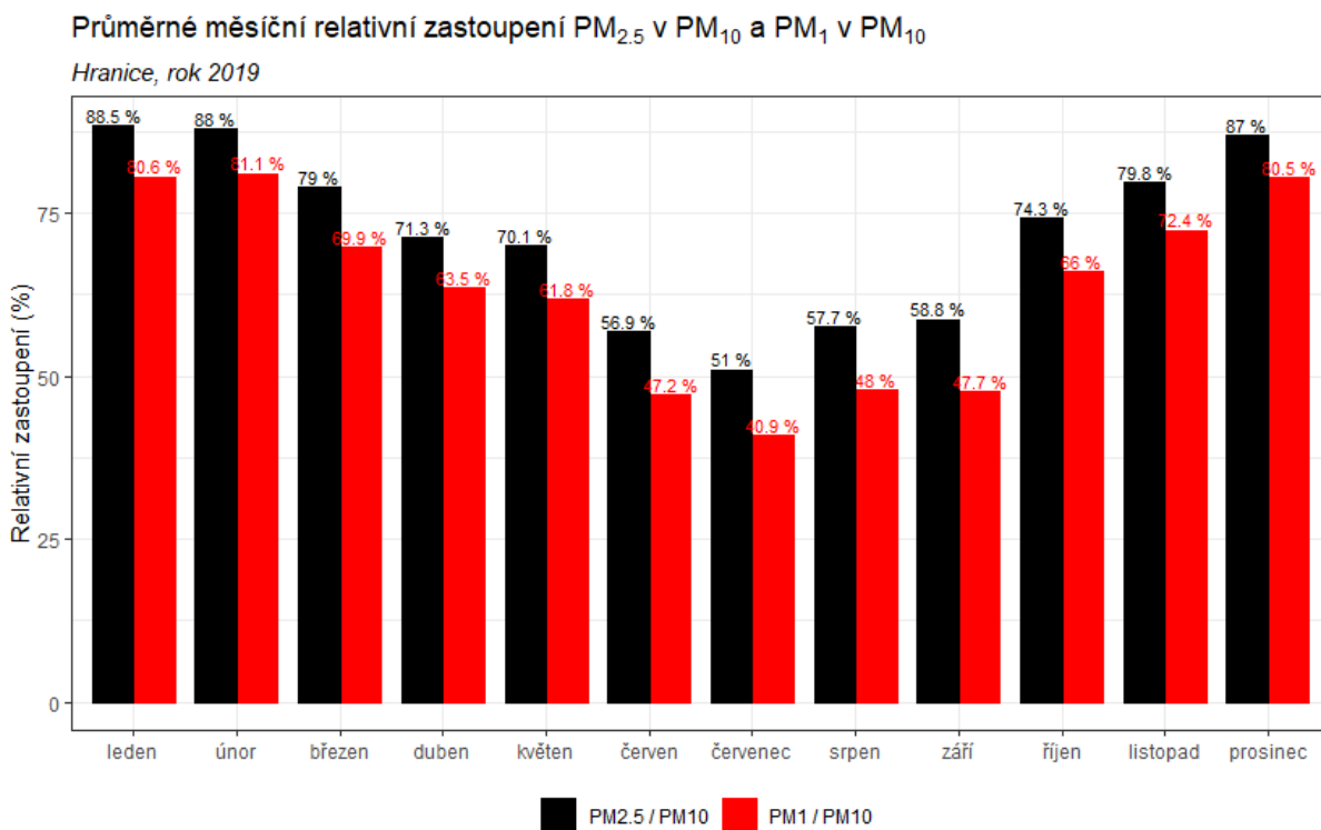
Obr. 19 – Průměrné měsíční zastoupení PM 2,5 v PM 10 a PM 1 v PM 10 , lokalita Hranice, rok 2019
