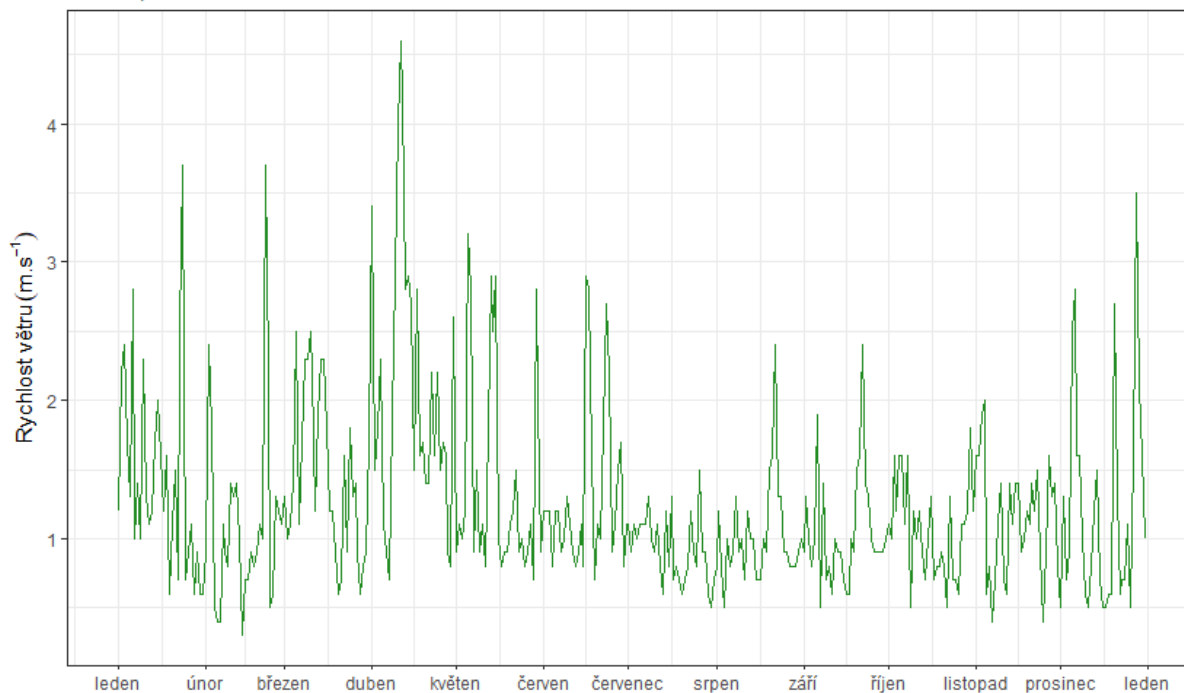
Obr. 2 – Průměrné denní rychlosti větru, Hranice, rok 2019
