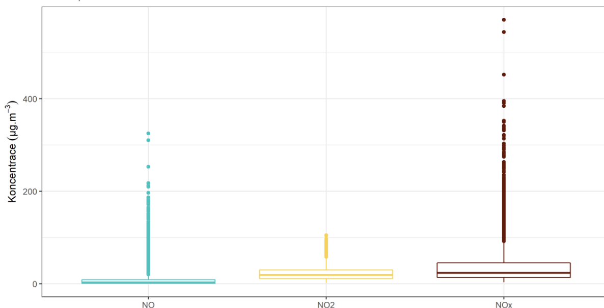
Obr. 39 – Statistické zpracování hodinových koncentrací NO, NO 2 a NO x v lokalitě Hranice, rok 2019
