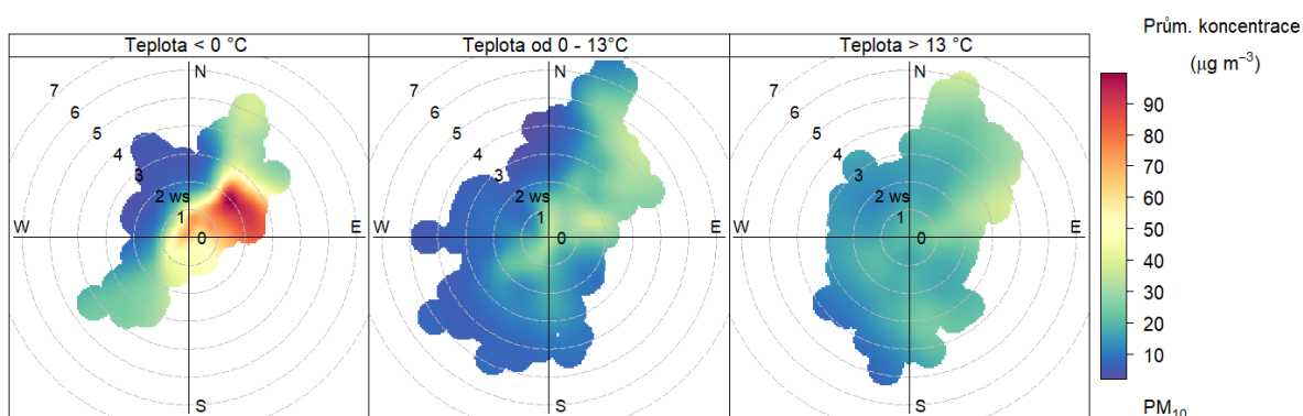
Obr. 30 – Koncentrační růžice členěná dle teplot, Hranice, rok 2019
