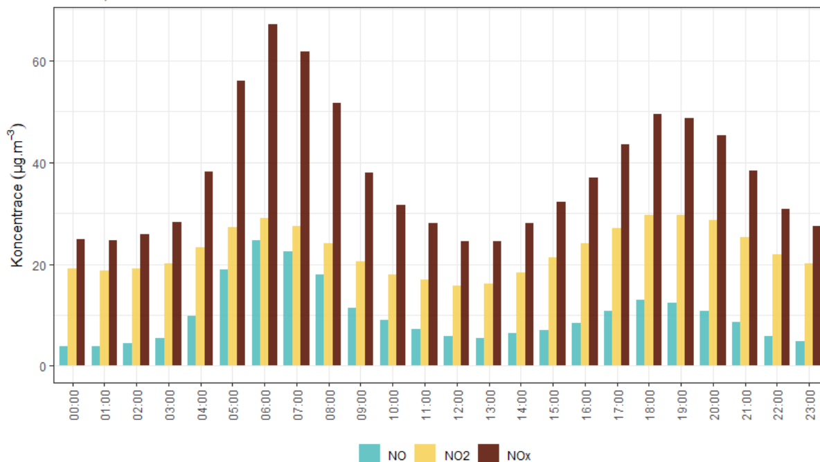
Obr. 45 – Denní chod hodinových koncentrací NO 2 , Hranice, rok 2019
