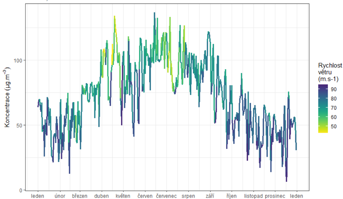
Obr. 58 – Vliv teploty (nahore) a rychlosti větru (dole) na koncentrace O 3 , Hranice, rok 2019
