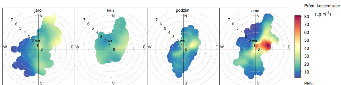
Obr. 29 – Koncentrační růžice jednotlivých ročních období, Hranice, rok 2019
