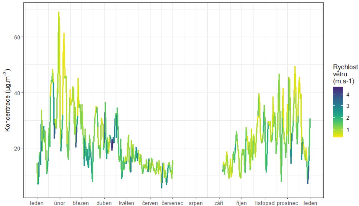
Obr. 43 – Vliv teploty (nahore) a rychlosti větru (dole) na koncentrace NO 2 , Hranice, rok 2019
