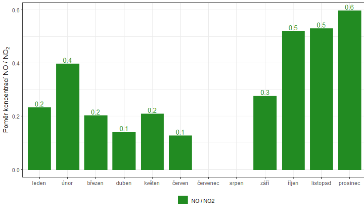
Obr. 41 – Poměr měsíčních koncentrací NO / NO 2 , lokalita Hranice, rok 2019
