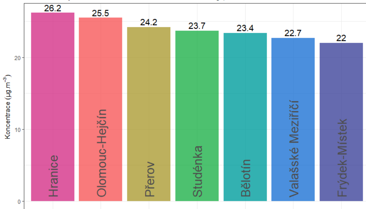
Obr. 32 – Srovnání průměrné roční koncentrace PM 10 lokality Hranice s okolními stanicemi státní sítě imisního monitoringu, rok 2019
