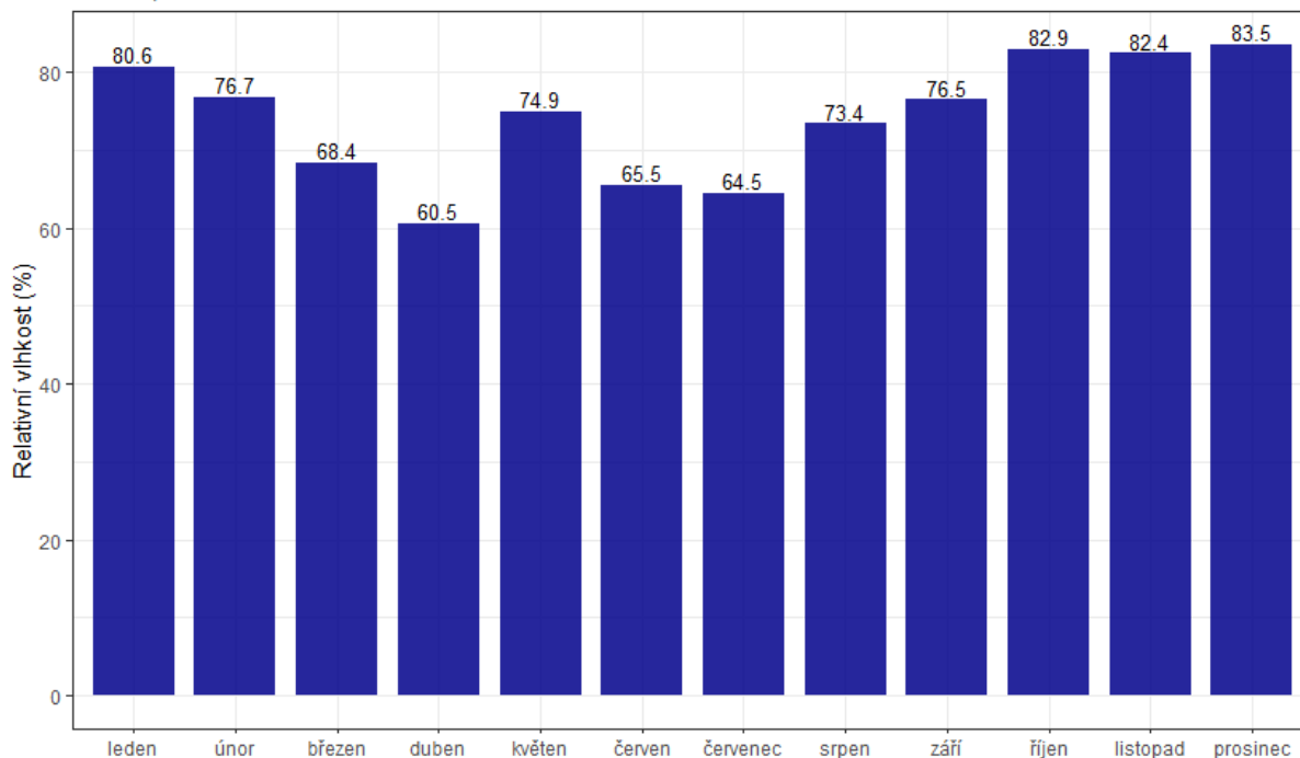
Obr. 7 – Průměrné měsíční relativní vlhkosti vzduchu, Hranice, rok 2019
